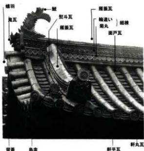
第6図 屋根瓦名称図 (森2001より転載)
