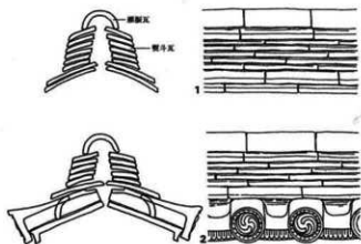
第7図 「棟」模式図 (上原2001に一部加筆)
