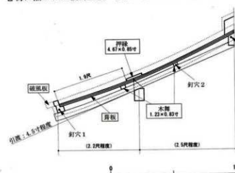
【図3】柳之御所遺跡出土部材にもとづく板葺屋根復元断面図
