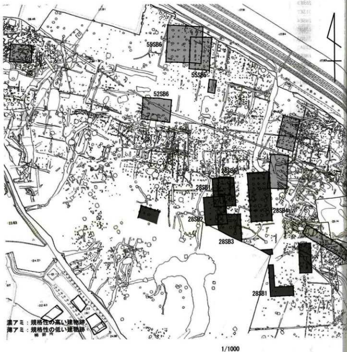
図4 柳之御所遺跡堀内部掘立柱建物の規格性
