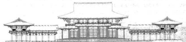
〔図14〕毛越寺復元立面図
