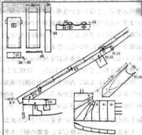
【図⑥】中尊寺金色堂木瓦詳細図
