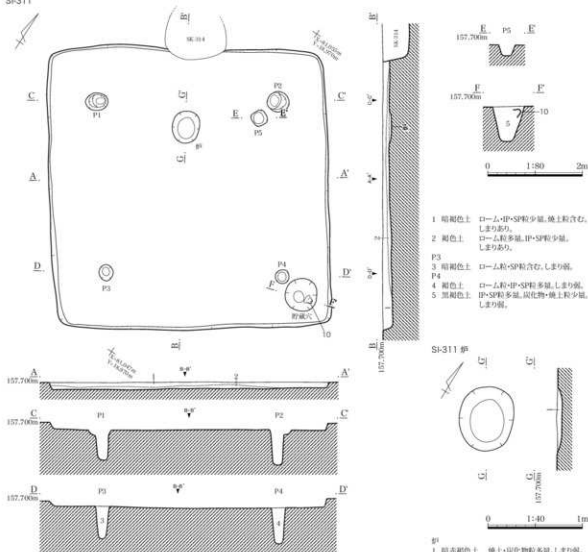
第34図 小鍋内I遺跡 SI-311 実測図
