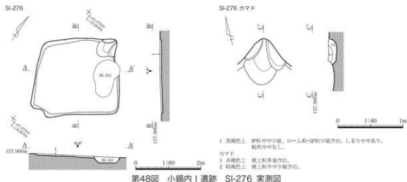
第48図 小鍋内I遺跡 SI-276 実測図
