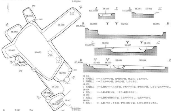
第79図 小鍋内I遺跡 中世以降土坑実測図(4)
