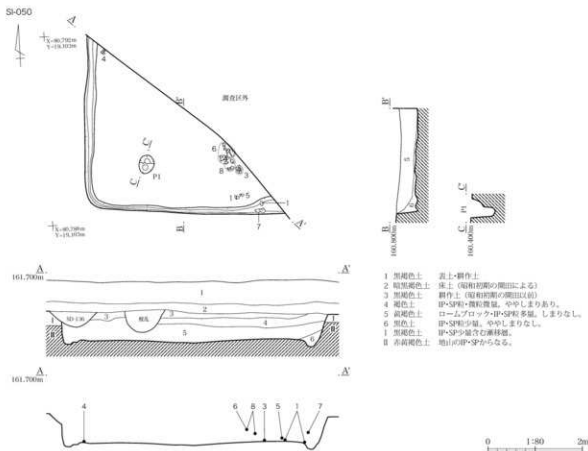
第134図 小鍋内Ⅱ遺跡 SI-050 実測図
