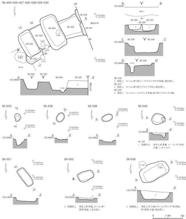
第216図 小鍋内Ⅱ遺跡 中世以降土坑実測図(15)
