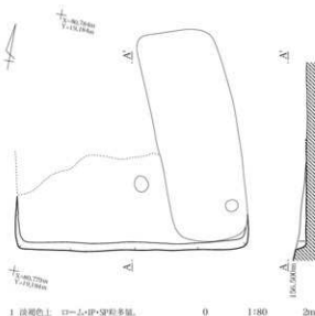
第153図 小鍋内Ⅱ遺跡 SI-301 実測図
