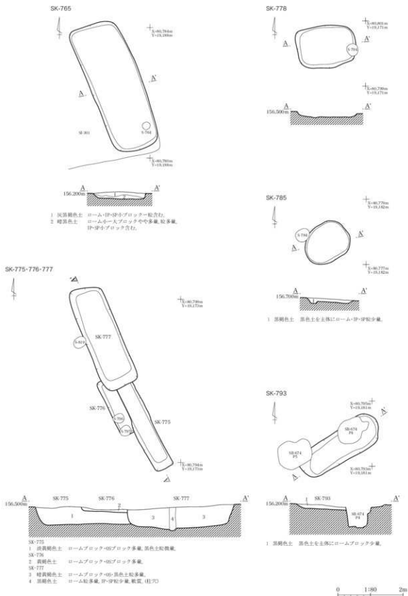
第227図 小鍋内Ⅱ遺跡 中世以降土坑実測図(21)
