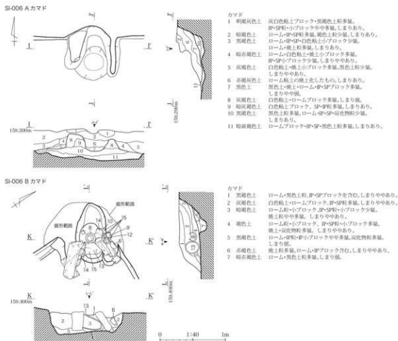
第127図 小鍋内Ⅱ遺跡 SI-006 実測図(2)
