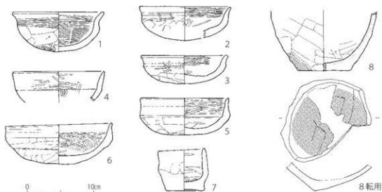
第133図 小鍋内II遺跡 SI-008 出土遺物実測図
