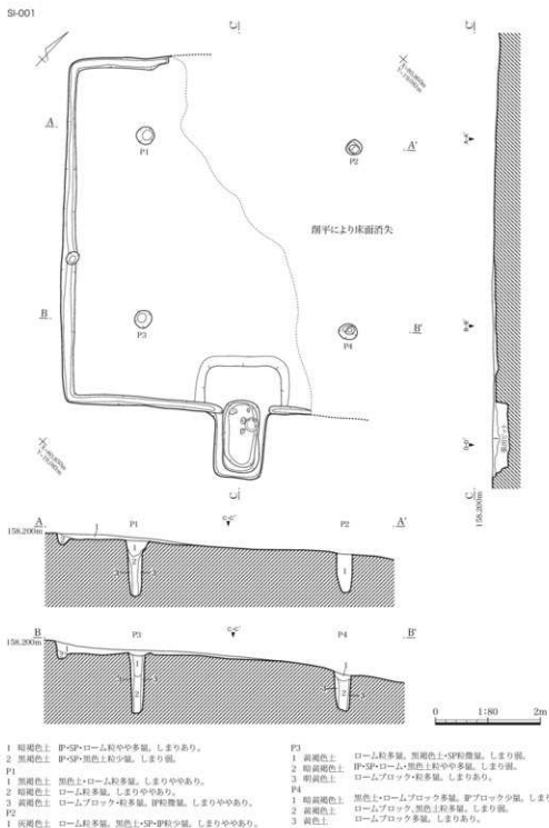
第117図 小銅内Ⅱ遺跡 SI-001 実測図(1)
