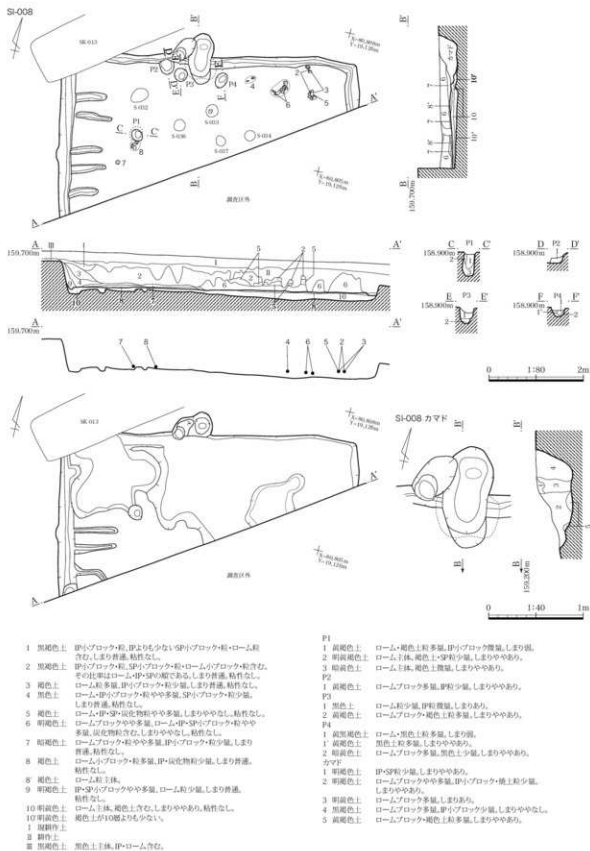
第132図 小鍋内Ⅱ遺跡 SI-008 実測図
