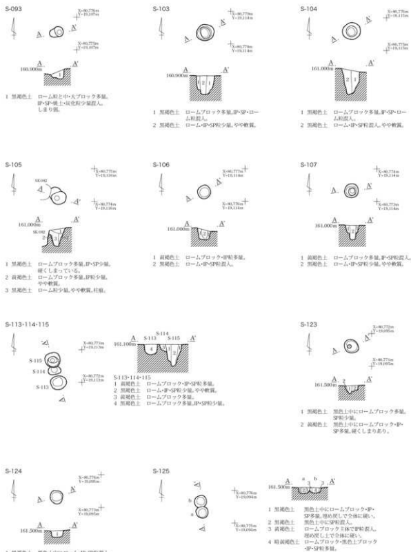
第232図 小鍋内Ⅱ遺跡 中世以降ピット実測図(1)
