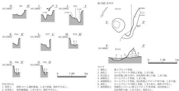
第178図 小銅内Ⅱ遺跡 SI-102 実測図 (2)
