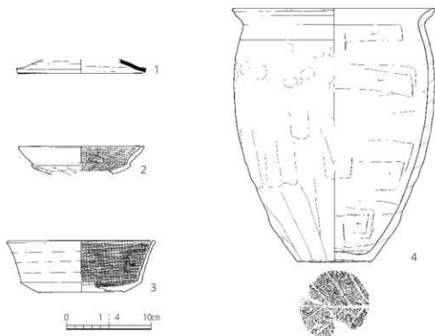
第189図 小鍋内Ⅱ遺跡 SI-303 出土遺物実測図
