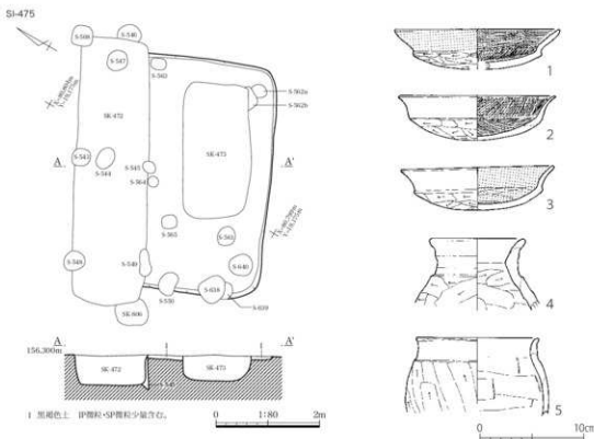
第155図 小鍋内Ⅱ遺跡 SI-475 実測図及び出土遺物実測図
