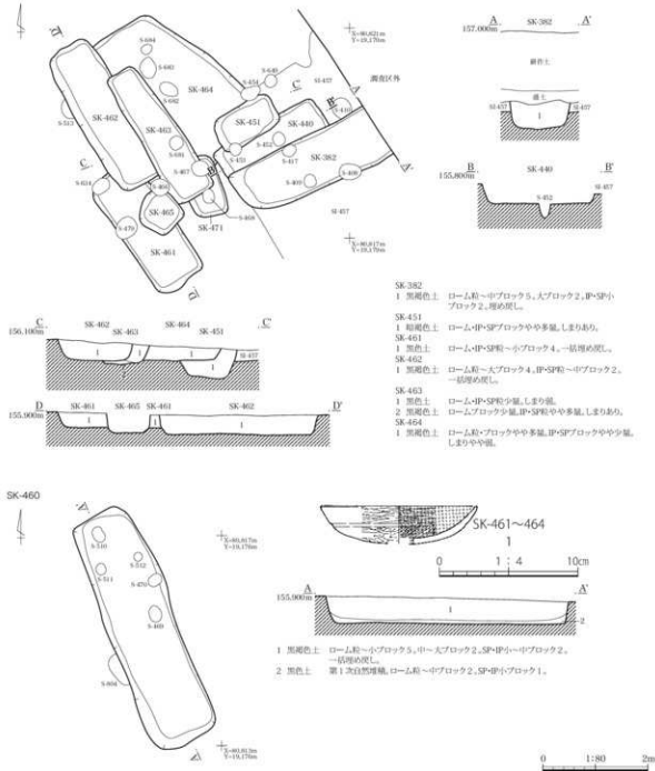
第211図 小鍋内Ⅱ遺跡 中世以降土坑実測図(12)及びSK-461～SK-464出土遺物実測図
