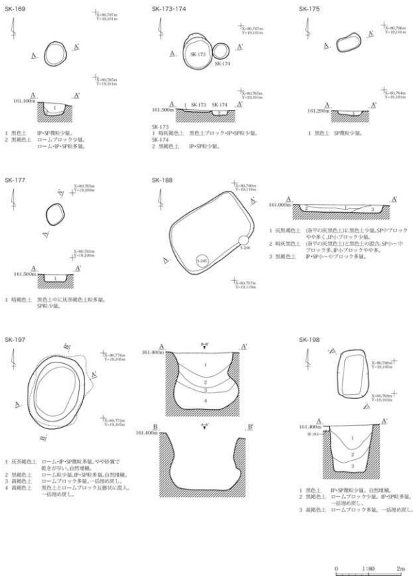
第204図 小鍋内Ⅱ遺跡 中世以降土坑実測図(6)
