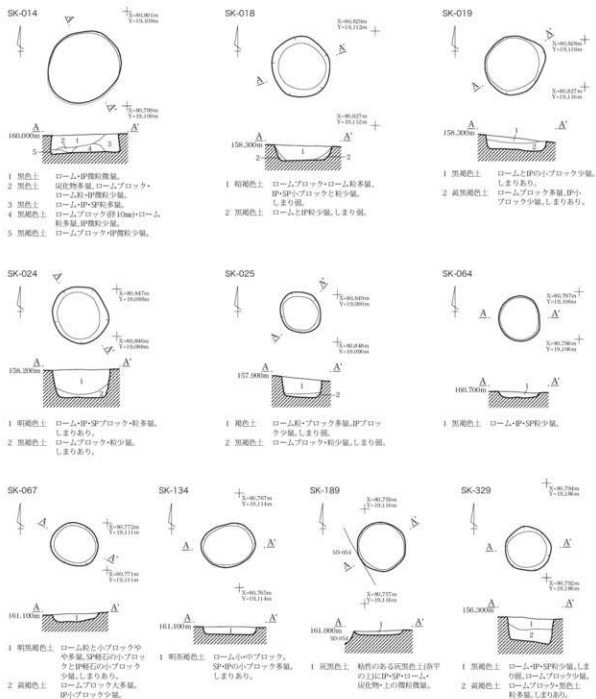
第158図 小鍋内Ⅱ遺跡 古墳時代土坑実測図
