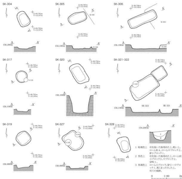
第206図 小鍋内Ⅱ遺跡 中世以降土坑実測図(8)
