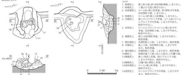
第140図 小鍋内II遺跡 SI-055 実測図
