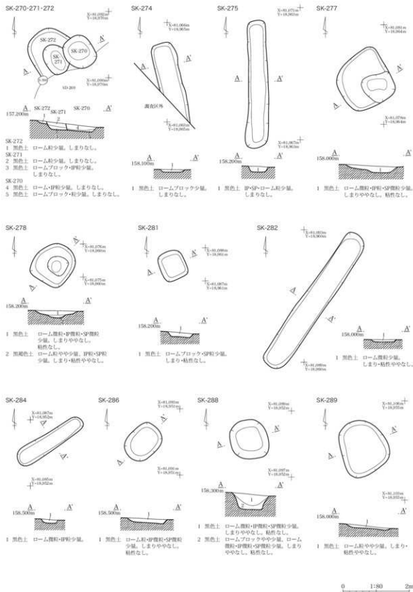
第94図 小銅内1遺跡 中世以降土坑実測図 (18)
