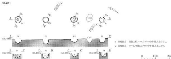
第162図 小鍋内Ⅱ遺跡 SA-821 実測図
