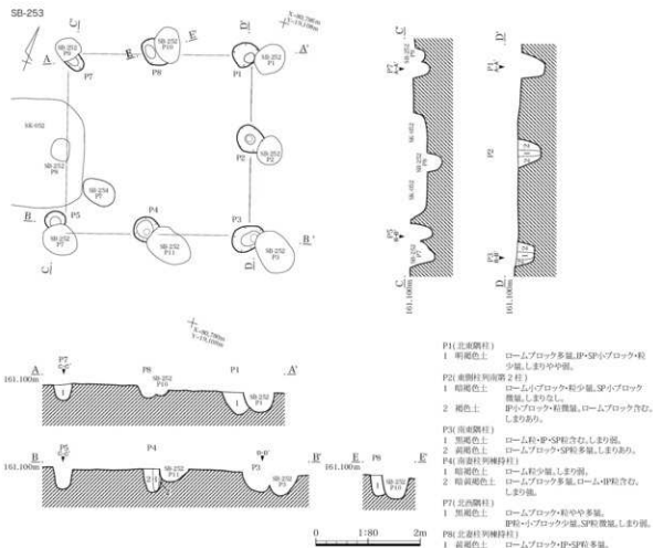
第168図 小鍋内Ⅱ遺跡 SB-253 実測図
