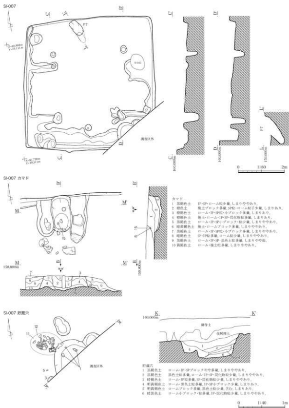
第130図 小銅内II遺跡 SI-007 実測図(2)
