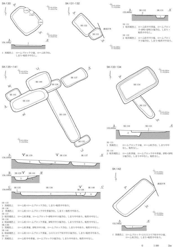
第84図 小鍋内I遺跡 中世以降土坑実測図(9)
