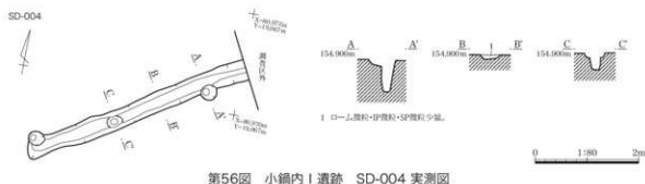
第56図 小鍋内I遺跡 SD-004 実測図
