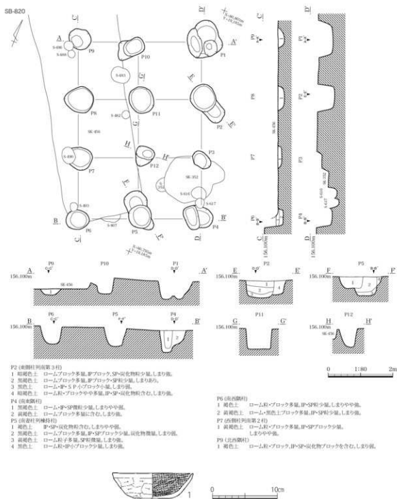
第174図 小鍋内Ⅱ遺跡 SB-820 実測図及び出土遺物実測図
