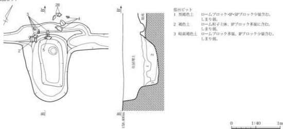
第120図 小銅内Ⅱ遺跡 SI-002 実測図(2)
