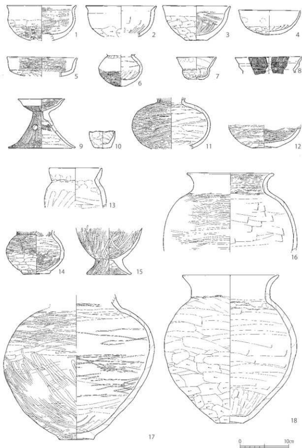
第23図 小銅内I遺跡 SI-299 出土遺物実測図
