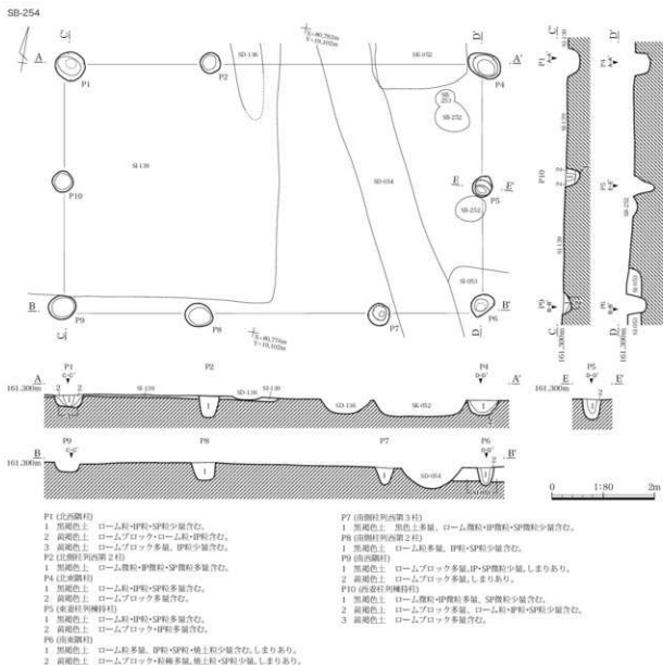
第169図 小鍋内Ⅱ遺跡 SB-254 実測図
