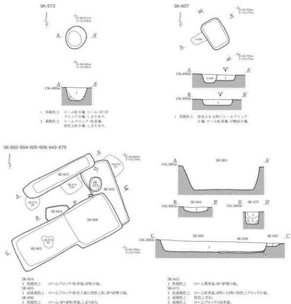
第224図 小鍋内Ⅱ遺跡 中世以降土坑実測図(19)
