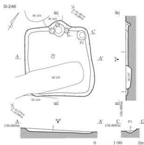
第46図 小竈内I遺跡 SI-246 実測図
