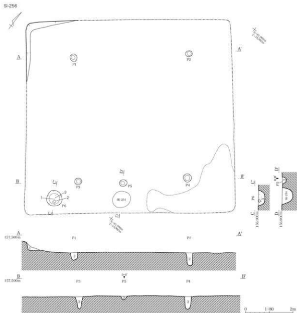
第16図 小鍋内I遺跡 SI-256 実測図
