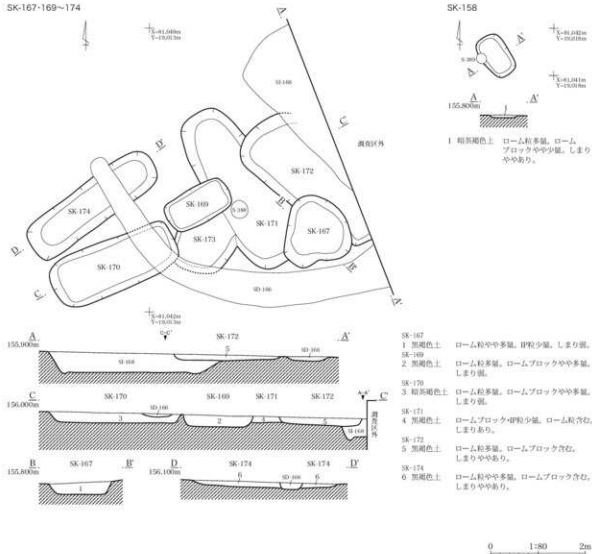
第86図 小鍋内I遺跡 中世以降土坑実測図(11)
