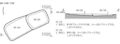
第85図 小銅内I遺跡 中世以降土坑実測図(10)
