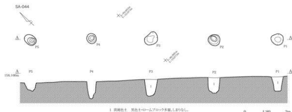
第161図 小鍋内Ⅱ遺跡 SA-044 実測図
