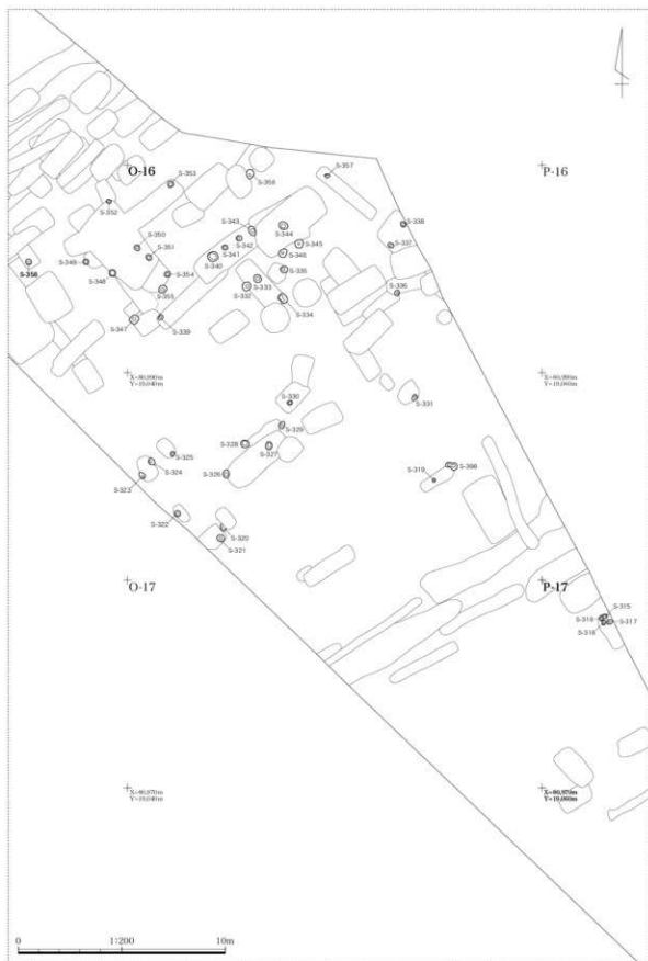
第100図 小銅内I遺跡 ビット分布図 (C)
