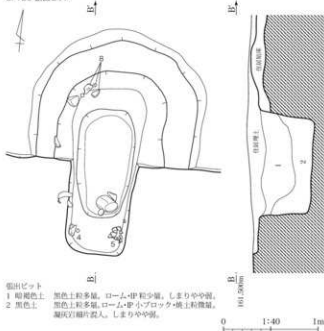
第149図 小鍋内Ⅱ遺跡 SI-185 実測図
