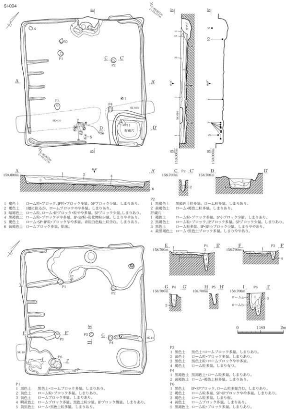
第123図 小鍋内Ⅱ遺跡 SI-004 実測図(1)
