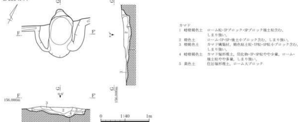
第151図 小鍋内Ⅱ遺跡 SI-300 実測図
