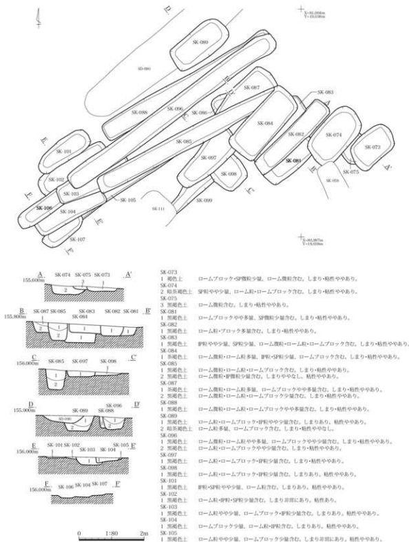
第82図 小鍋内I遺跡 中世以降土坑実測図(7)
