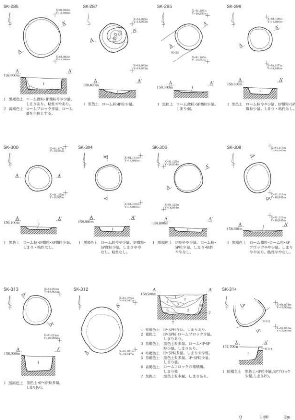
第39図 小鍋内I遺跡 古墳時代土坑実測図(2)
