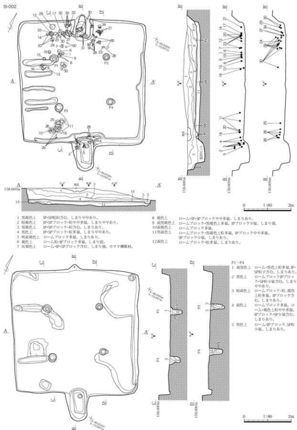
第119図 小銅内Ⅱ遺跡 SI-002 実測図(1)
