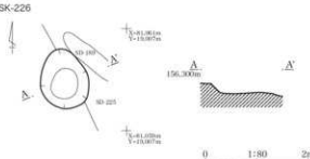
第91図 小鍋内I遺跡 中世以降土坑実測図 (15)
