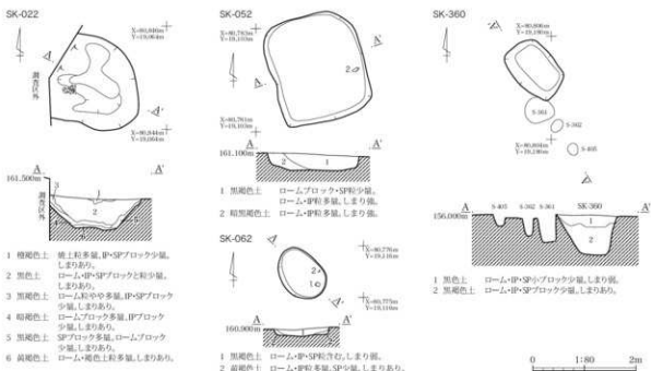
第190図 小鍋内Ⅱ遺跡 奈良・平安時代土坑実測図
