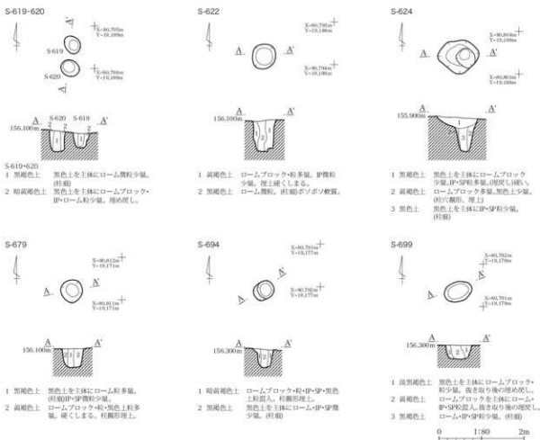
第235図 小鍋内Ⅱ遺跡 中世以降ピット実測図(3)
