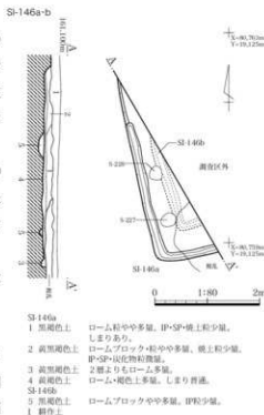
第146図 小鍋内Ⅱ遺跡 SI-146 実測図
