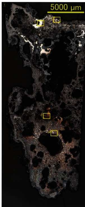
Photo.3 鉄塊系遺物の顕微鏡組織
