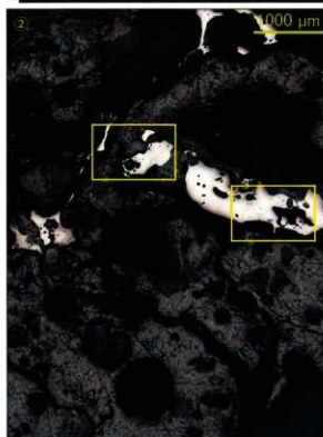
Photo.7 梶形鍛冶滓の顕微鏡組織
