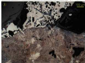
Photo.1 鉄塊系遺物の顕微鏡組織
