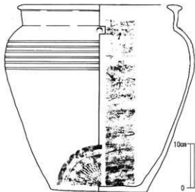
第17図 N G 84-3 次襲実測図
