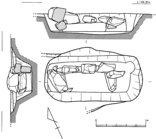
第14図 NG84-2次SX-01実測図
