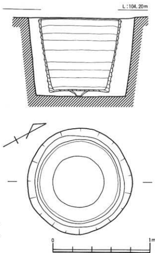
第10図 NG84-2次埋壘-02実測図
