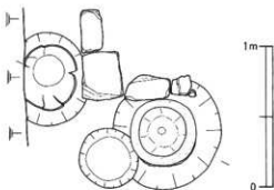
第16図 N G 84-3 次埋襲・手水鉢実測図
