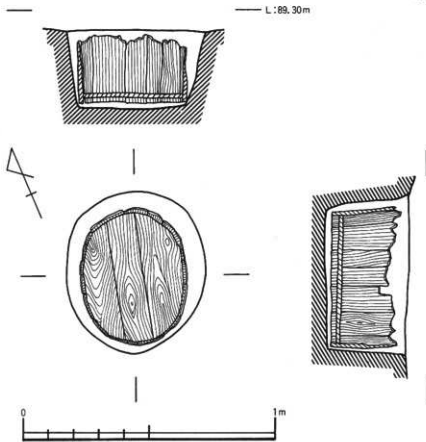
第5図 NG84-1 次埋桶-02実測図
