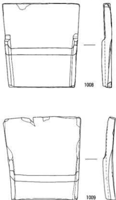
第13図 NG84—2次瓦列瓦実測図
