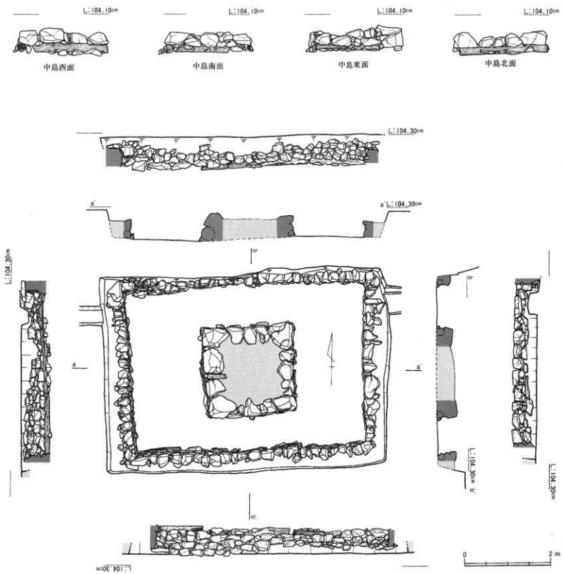
第11図 NG84-2次SG-01実測図
