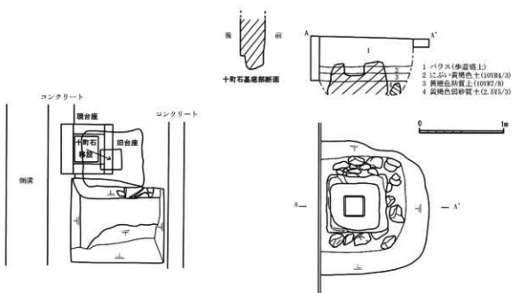
十町石と旧台座の平面位置図 (S=1/40)
