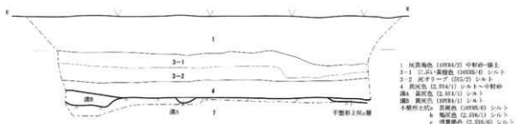
1トレンチ 平面図・土層断面図 S=1/50
