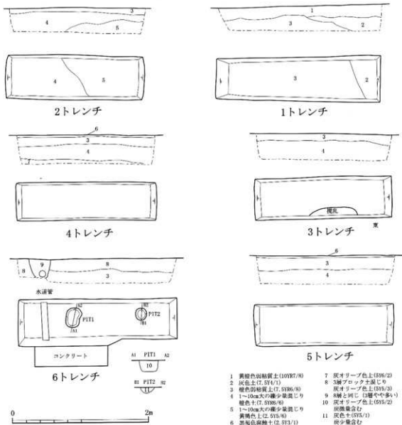
トレンチ平面図・土層断面図 (S=1/40)
