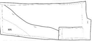
2トレンチ平面図・土層断面図 S=1/60
