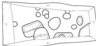
8トレンチ平面図・土層断面図 S=1/60
