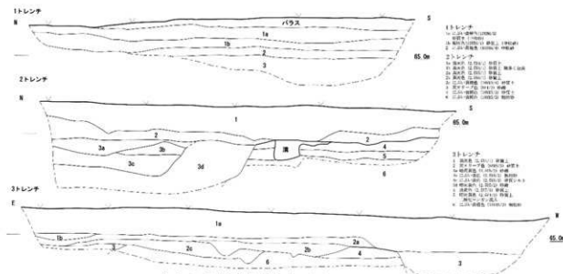
トレンチ土層断面図 (S=1/50)
