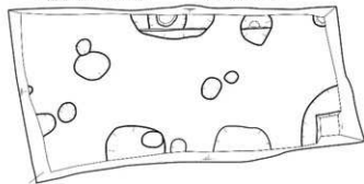
6トレンチ平面図・土層断面図 S=1/60
