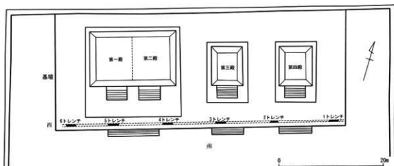
調査位置図 (S=1/500)
