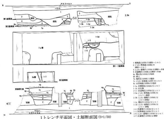
1トレンチ平面図・土層断面図 (S=1/50)
