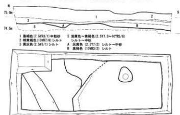
18トレンチ平面図・土層断面図 S=1/60
