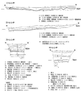
トレンチ土層断面図 S=1/80
