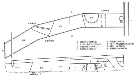
C区 平面図・土層断面図 S=1/60
