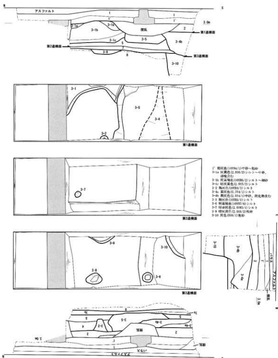
3トレンチ 平面図・土層断面図 (S=1/50)
