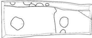
7トレンチ平面図・土層断面図 S=1/60
