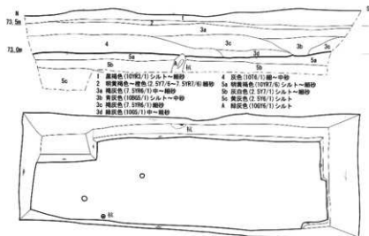
20トレンチ平面図・土層断面図 / S=1/60
