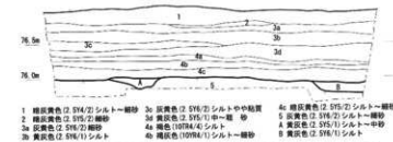
15トレンチ平面図・土層断面図 S=1/60
