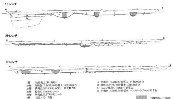
トレンチ土層断面図 S=1/80
