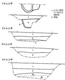
トレンチ土層断面図 S=1/50
