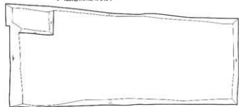
12 トレンチ平面図・土層断面図 S=1/60
