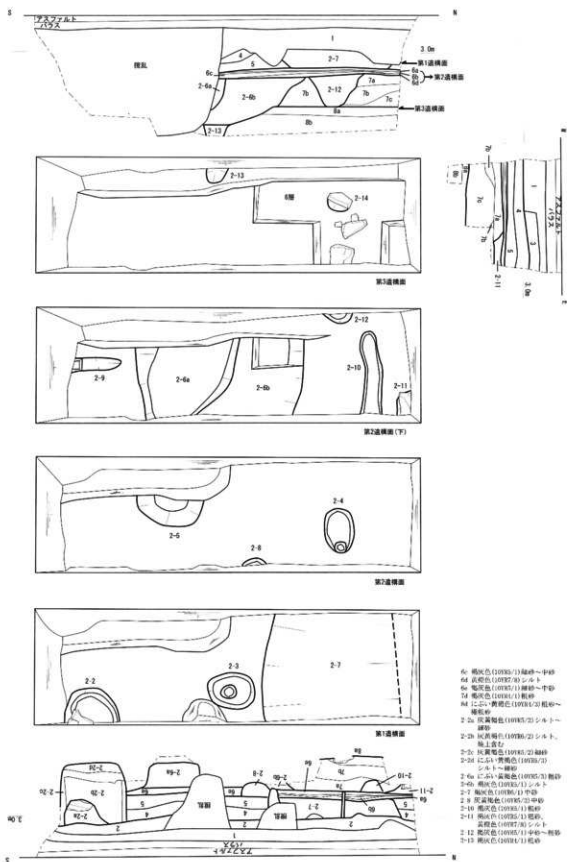
2トレンチ 平面図・土層断面図 (S=1/50)
