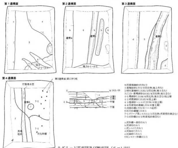
2グリッド平面図及び断面図 (S=1/60)
