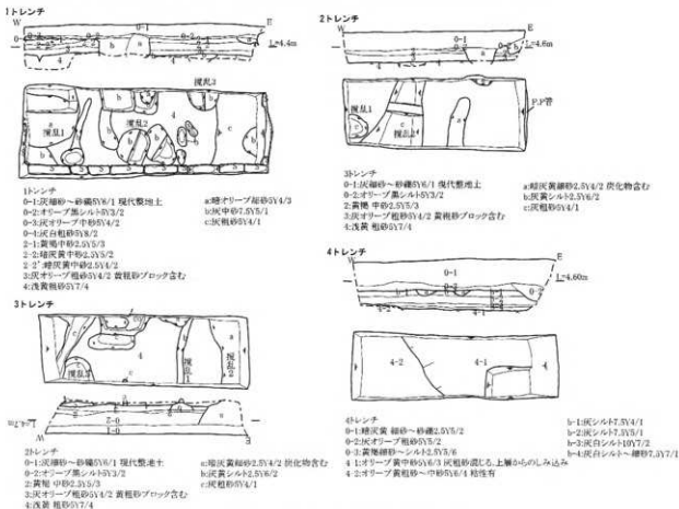
トレンチ平面図及び断面図 (S=1/100)
