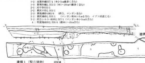
府中IV遺跡工事立会平面図及び断面図 1 (S=1/80)
