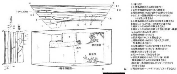
平面図・断面図(S=1/100)
