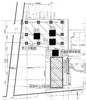
調査位置図 (S=1/800)
