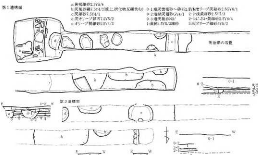
No.5 工事立会平面図・断面図 (S=1/40)
