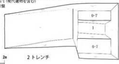
平面図・断面図① (S=1/100)
