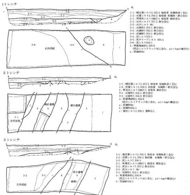
工事立会1~3トレンチ平面図及び断面図 (S=1/80)
