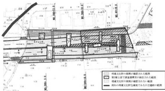
都市計画道路西脇山口線道路建設事業に伴う川辺遺跡埋蔵文化財取扱い図 (S=1/1,000)
