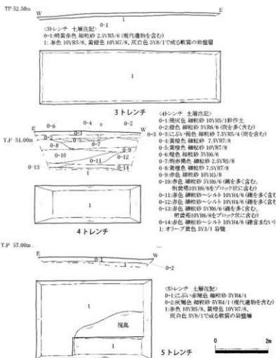
平面図・断面図②(S=1/100)
