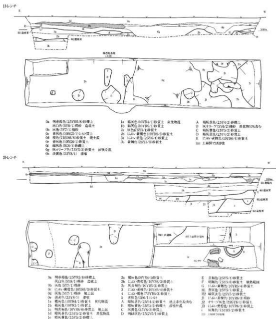
トレンチ平面図・土層図 S-1/80
