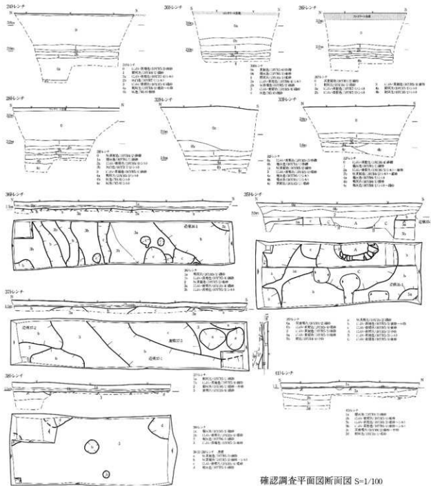
確認調査平面図断面図 S=1/100
