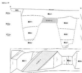
トレンチ平面図・断面図 S=1/100
