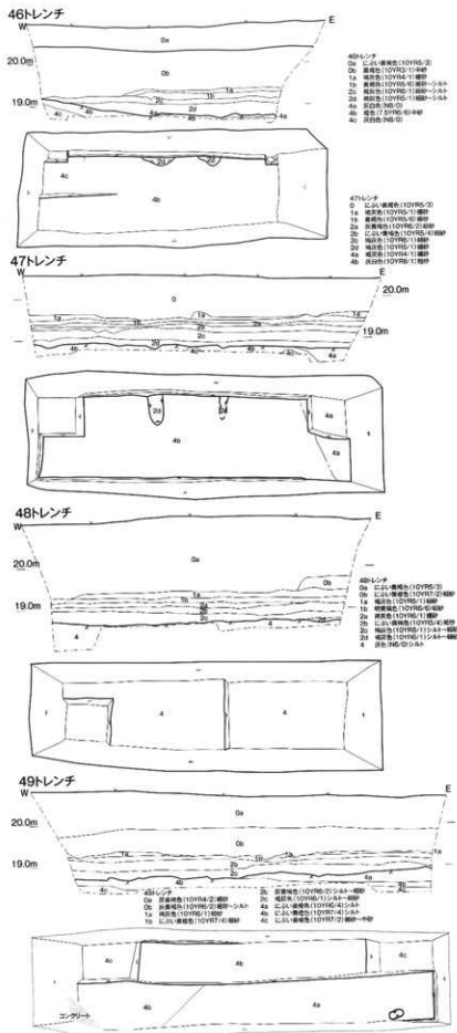
トレンチ平面図・断面図(S=1/100)
