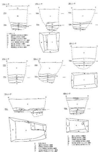
トレンチ平面図・断面図 S=1/100
