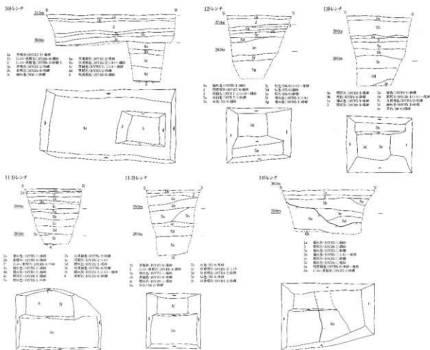
トレンチ平面図・断面図 S-1/100
