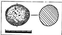
第8図 第4トレンチ出土石製投弾実測図
