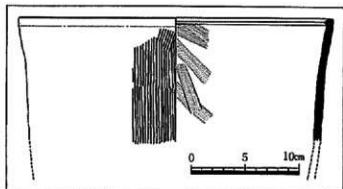
第9図 土師質観実測図
