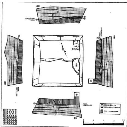
圖三十一 廣式之八輪船墓・墓室剖面圖
