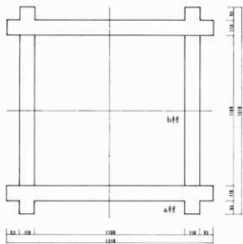
A型 平面
