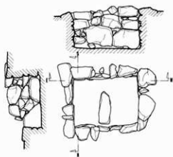
石構施設 SF 578 平面図・立面図
