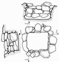
石構施設 SF 579 平面図・立面図
