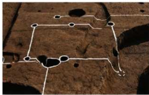
1 E区第6号掘立柱建物跡
