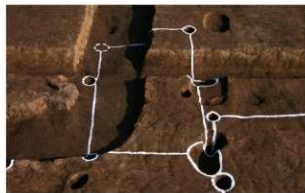
2 E区第7号掘立柱建物跡
