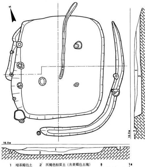
第10図 竪穴式建物SB04実測図 1/40
