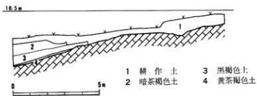
第7图 発掘区東壁土層図 1/150
