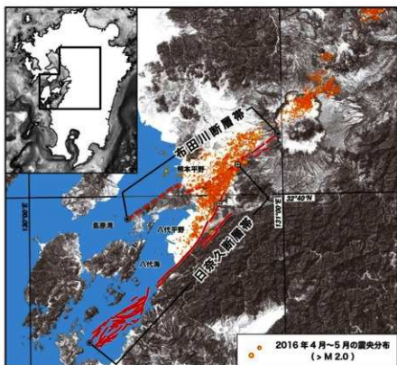
図1. 布田川断層・日奈久断層と2016年熊本地震に関係した地震の発生地点 布田川断層・日奈久断層は地震調査研究推進本部地震調査委員会(2013)による。
