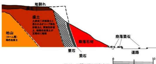
図11 百間石垣断面想定図
