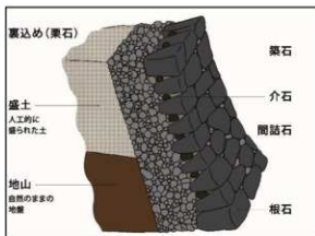
図 12 石垣構造概念図
