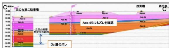
図9 C-C'地質断面図 (2019 中田)
