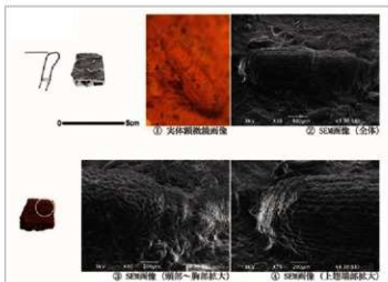
コクゾウムシ圧痕(三本松遺跡)
