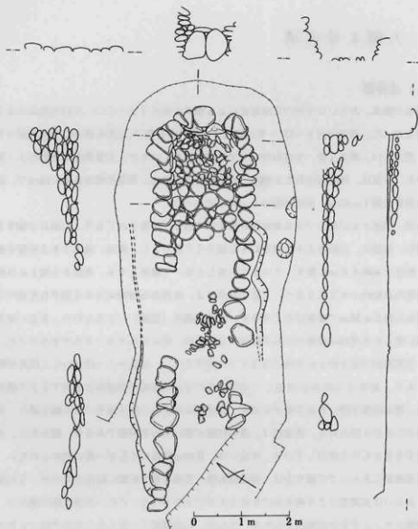
第4図 石室実測図
