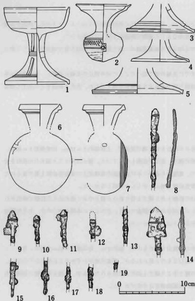
第5図 八幡4号古墳遺物実測図
