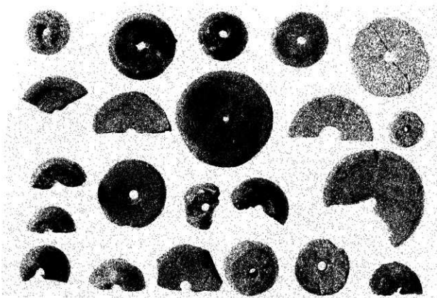
IX 紡錘車 (1)
