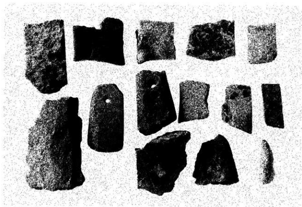
IX 礮石 (4)
