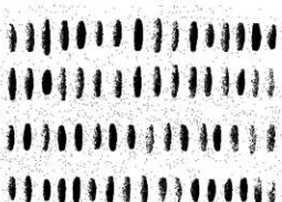
IX 土鍾 (4)
