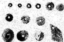
IX 土錘 (8)
