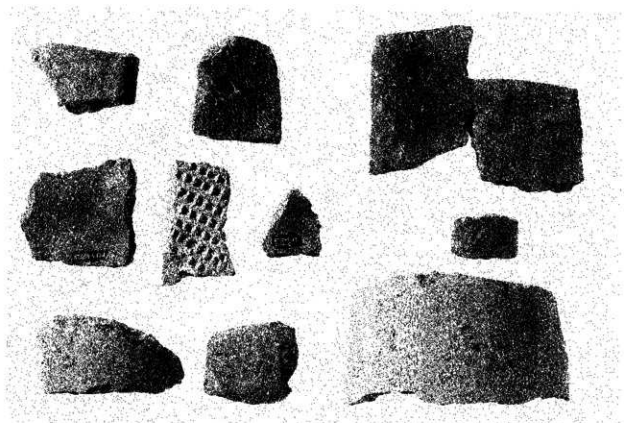
IX 瓦(3)裏
