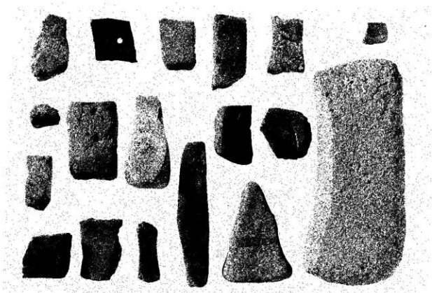
IX 礮石 (3)
