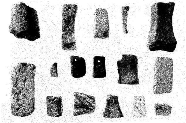
IX 礮石 (5)
