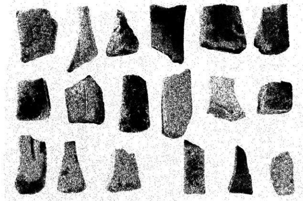
IX 礮石 (6)
