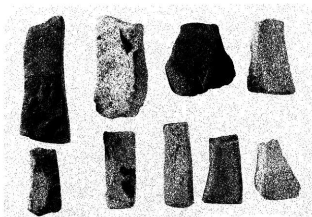
Ⅹ 礮石 (2)
