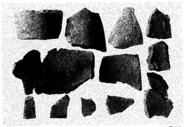
IX 瓦(1)
