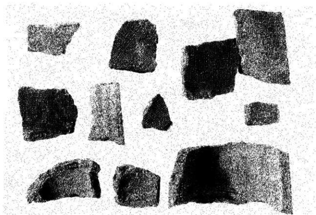
IX 瓦(2)表
