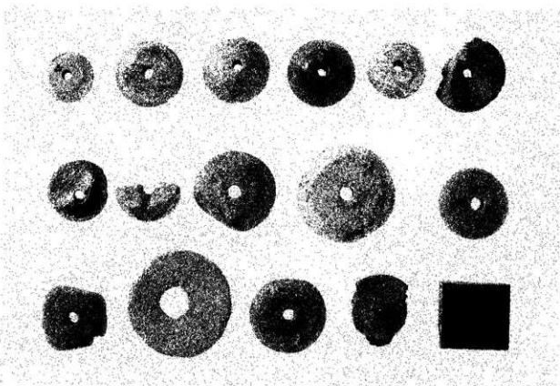
IX 紡錘車 (2)
