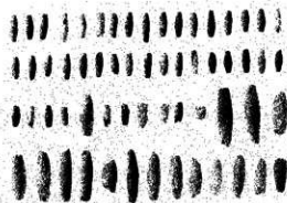
IX 土錘 (9)
