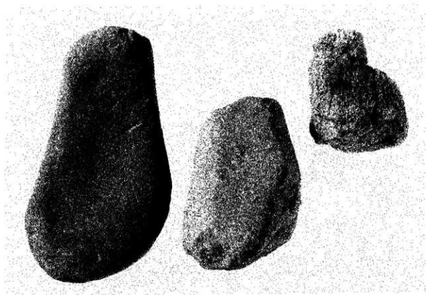
Ⅹ 礮石 (1)
