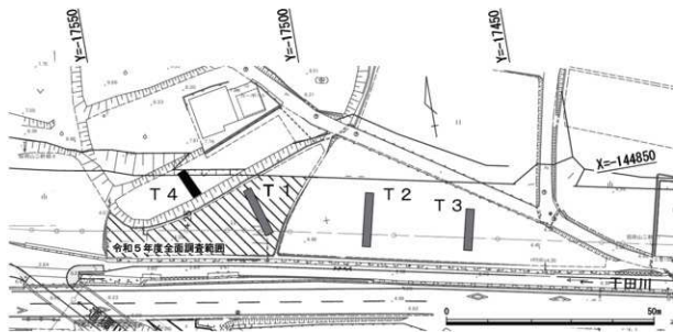
トレンチ配置図 (1/1,000)
