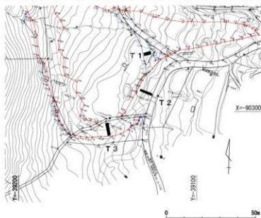
トレンチ配置図 (1/1,500)
