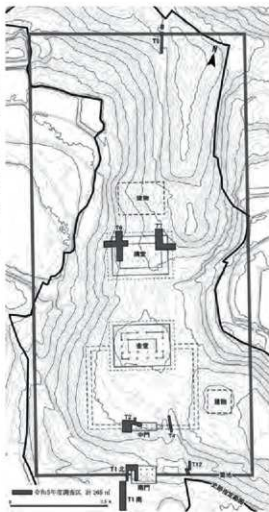
備中国分尼寺跡調査区配置図 (1/2,000)
