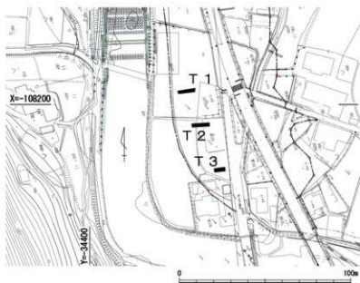
トレンチ配置図 (1/2,000)
