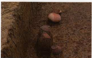
3 第 229 号住居跡遺物出土狀況 (2)
