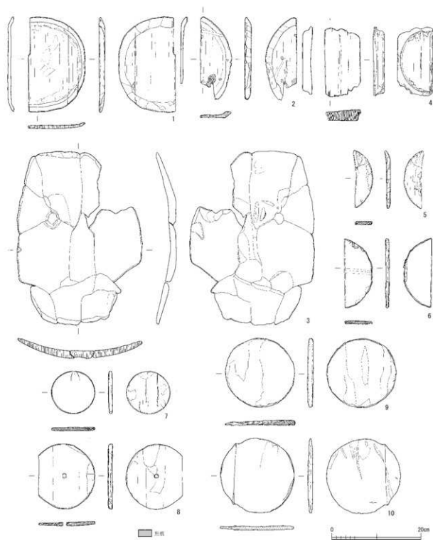
第22図 遺物実測図14 (縮尺1/6)
