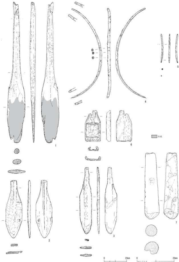
第21圖 遺物実測図13 (縮尺 1~4 : 1/10、5~7 : 1/6)
