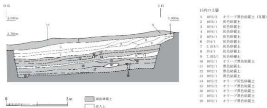
第6図 15列土層断面実測図(縮尺1/60)
