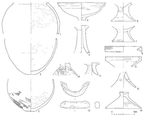
第17図 遺物実測図9 (縮尺1/4)
