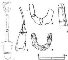
図3 U字形クワ・スキ先の柄と県内の類例
