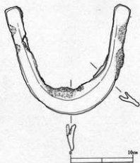
図2 U字形クワ・スキ先実測図
