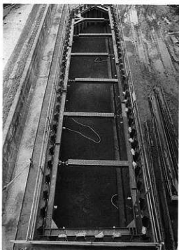
写真10 第V-2遺構面
