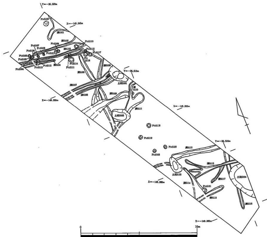
図15 第V-1 透視面透視尖刺図 (S=1/100)
