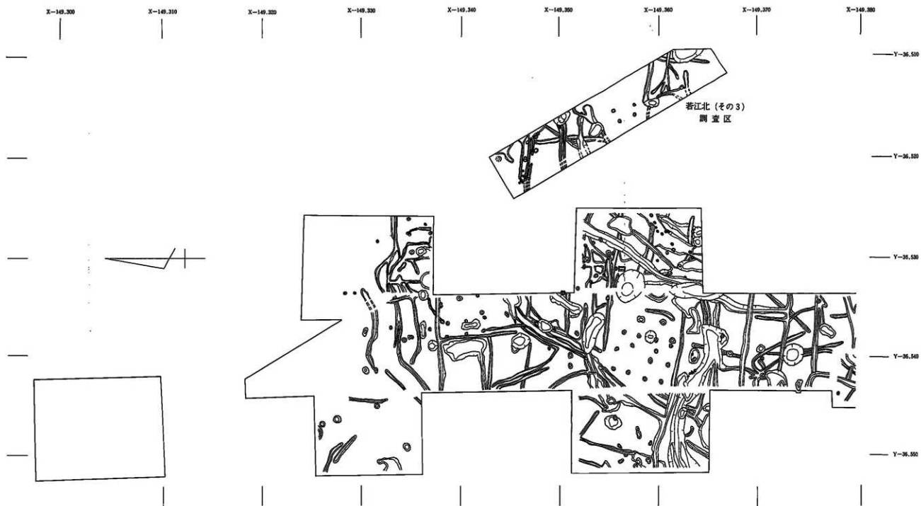
図14 第Y-1 透視面 透視配置図
