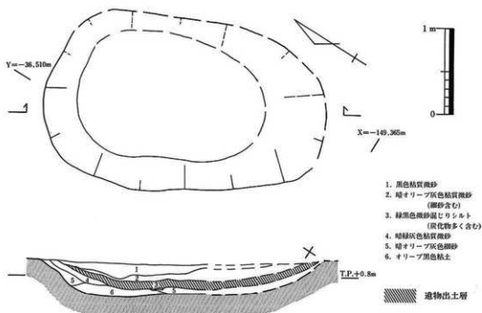
図16 土坑5104平面・断面図
