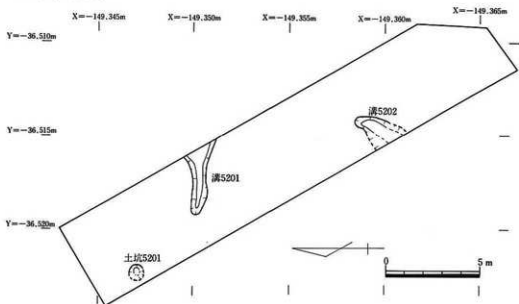
図20 第V-2遺構面遺構配置
