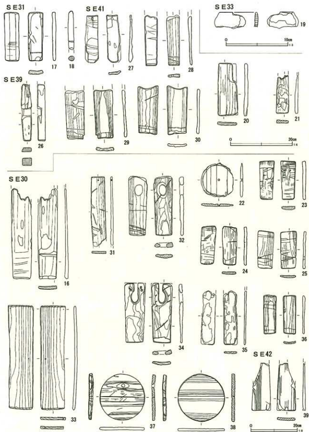
第216図 井戸跡出土木製品(2)
