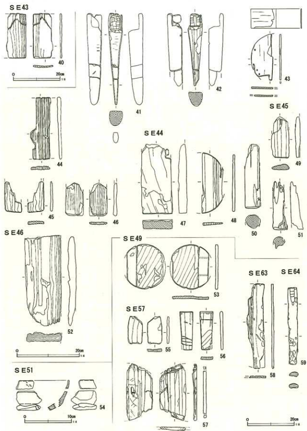
第217図 井戸跡出土木製品 (3)
