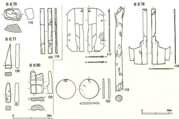
第222図 井戸跡出土木製品(8)
