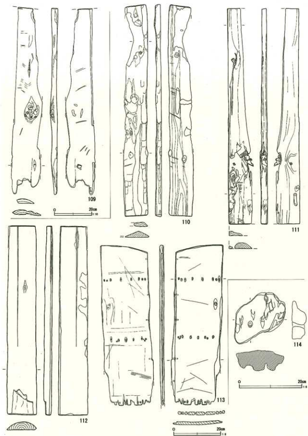
第221图 井戸跡出土木製品(7)
