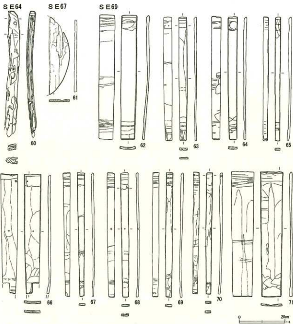
第218図 井戸跡出土木製品 (4)
