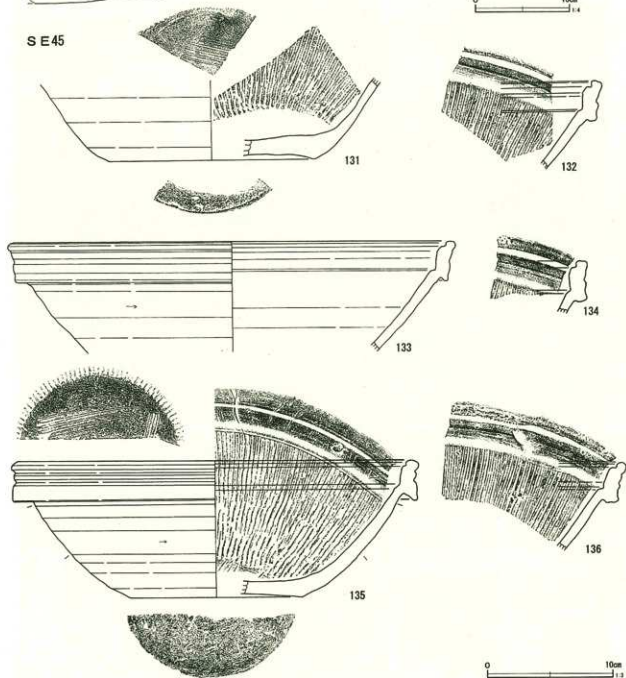
第211図 井戸跡出土遺物 (9)
