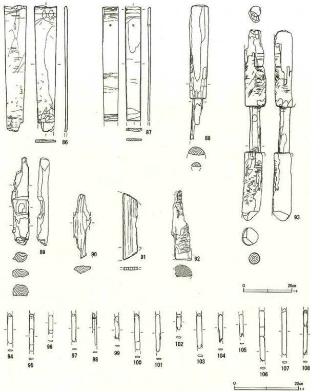
第220図 井戸跡出土木製品 (6)
