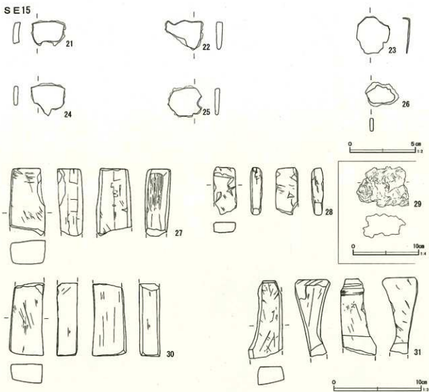
第204図 井戸跡出土遺物(2)
