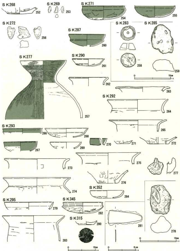
第189図 土城出土遺物 (10)
