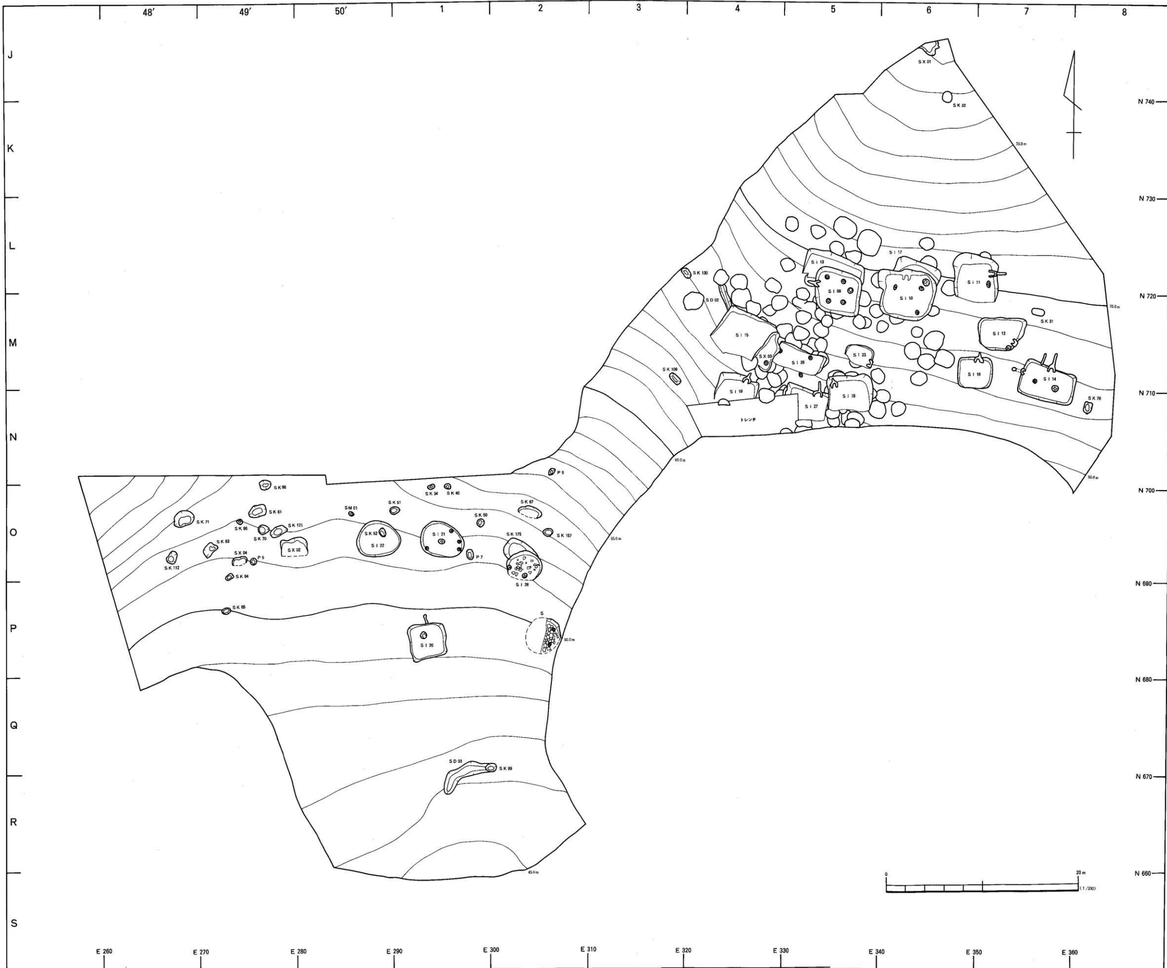
付図2 I区遺構配置図
