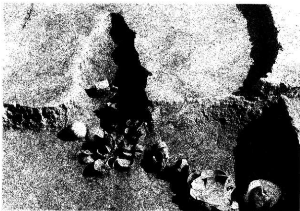
第297号住居跡カマド遺物出土状況
