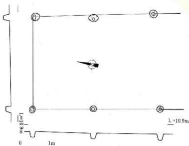
第28図 甲斐本C区1号掘立柱建物跡実測図 (1/80)
