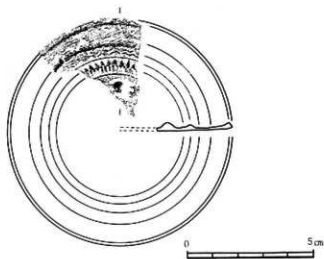
第23图 甲斐本B区出土鍍片实测图(2/3)
