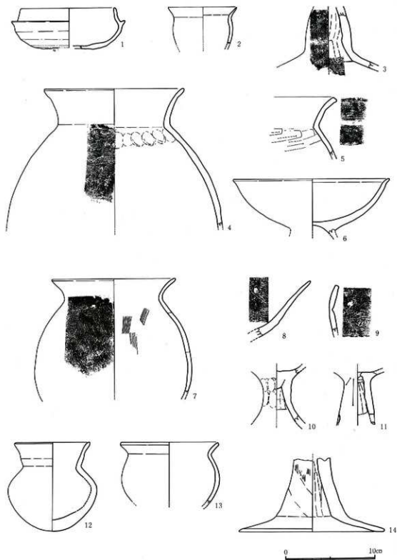
第19图 甲斐本A区出土遺物実測図1 (1/3)
