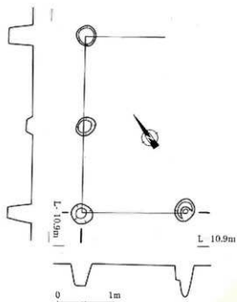
第24图 甲斐本B区1号獨立柱建物跡实测图(1/60)
