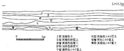
第3図 上戸原地区基本土層図(1/40)
