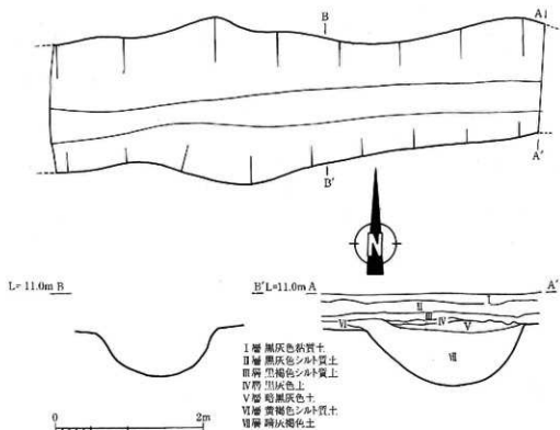
第6図 溝1平面・断面・土層実測図(1/60)
