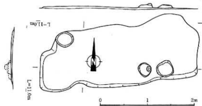
第5図 不整形土坑実測図(1/40)
