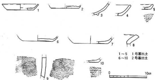
第9図 1号墓・2号墓出土遺物実測図
