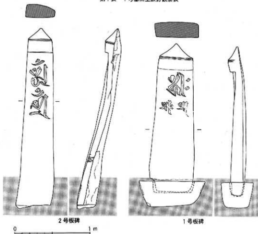
第11図 1号板碑・2号板碑実測図
