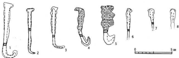
第10図 1号墓出土鉄釘実測図
