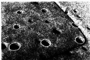
第37号掘立柱建物跡
