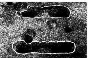
第35号掘立柱建物跡
