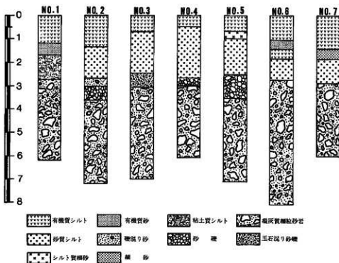
第 6 図 中曾根遺跡の主要地点柱状図
