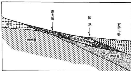
第4図 遺跡地質構造模式図
