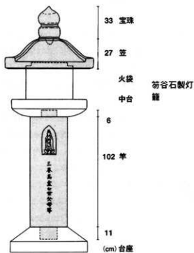
挿図2 石灯籠模式図
