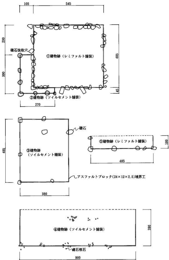
第11図 整備建物寸法図
