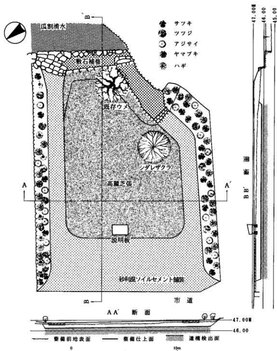
第9図 第106次調査瓜割流整備図
