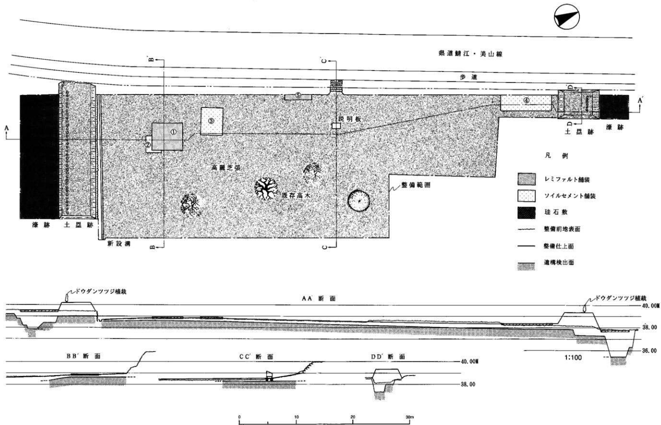
第10図 第68次調査中惣整備図
