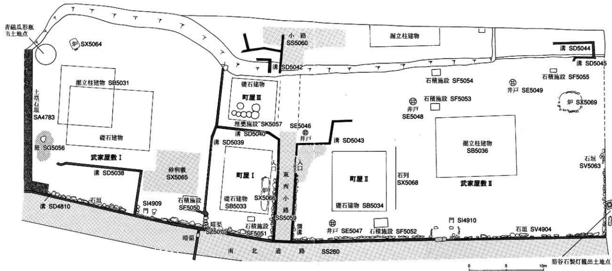
第4図 第112次発掘調査遺構模式図
