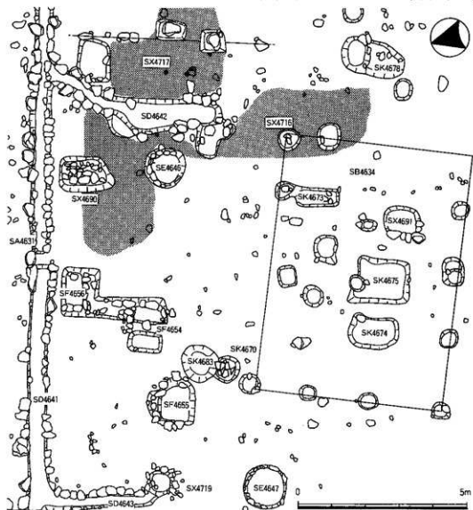
第3図 第100次調査遺構図(1)
