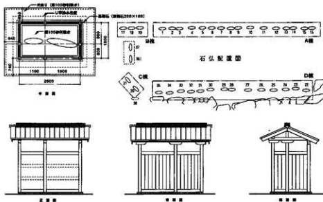
第15図 C棟平面・立面図
