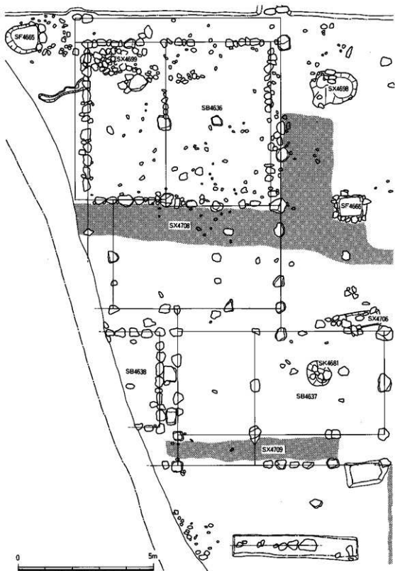
第6圖 第100次調査遺構図(4)
