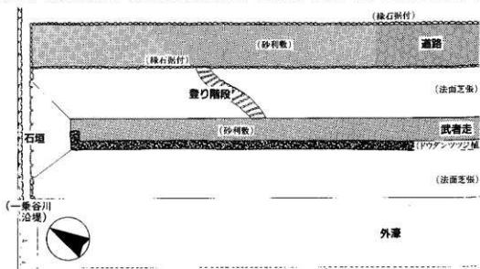
第29図 上城戸土塁復原整備工全体図 (1/400)
