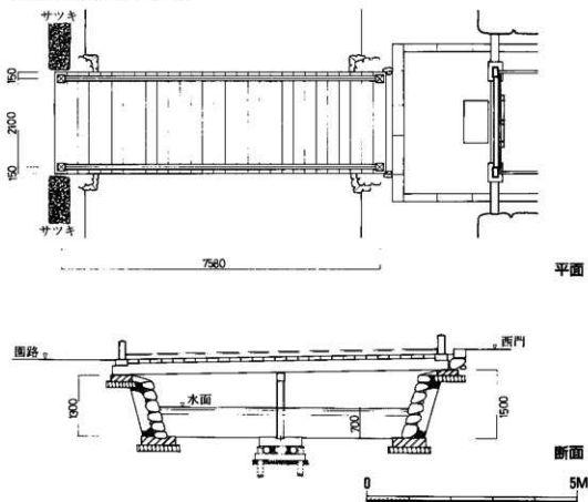
第31図 木製橋設計図(1/100)
