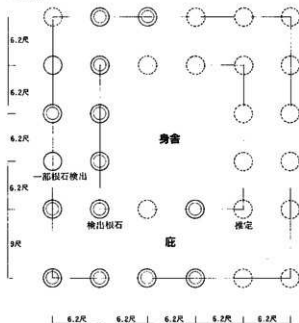
第6図 根石建物SB3722推定図
