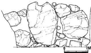
第4図 石垣S V 3712立面図
