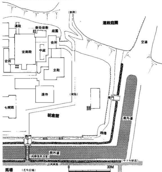
第30図 朝倉館外濠復原整備工全体図 (1/800)
