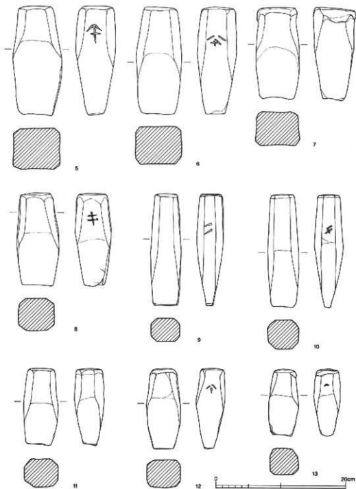
第18図 採石道具実測図(2)
