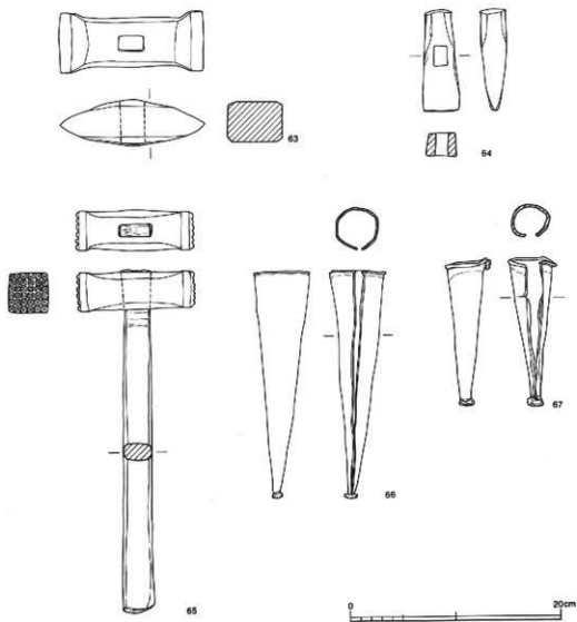
ハゲンノウ(63・64) ビシャン(65) カネツツ(66-67)
