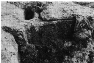
第14図 加茂山No15地点矢穴細部
