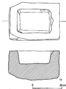
第26図 採石道具実測図(10) ミズイレ
