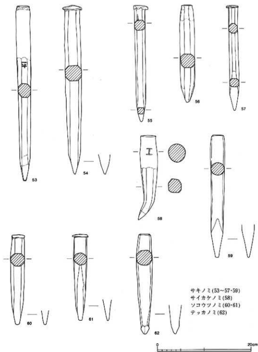
第23図 採石道具実測図(7)
