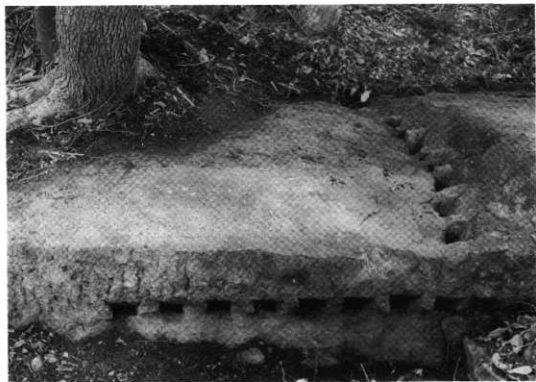
竜山石切場跡 00-1地点 矢穴
