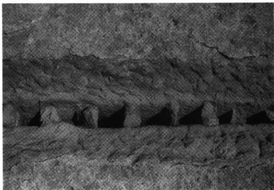
竜山石切場跡 I H-14地点 矢穴
