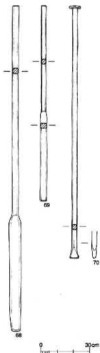
第25図 採石道具実測図(9)
