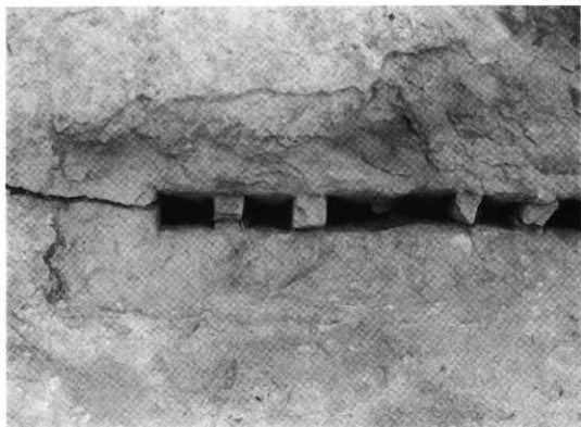
竜山石切場跡 KA-25地点 矢穴
