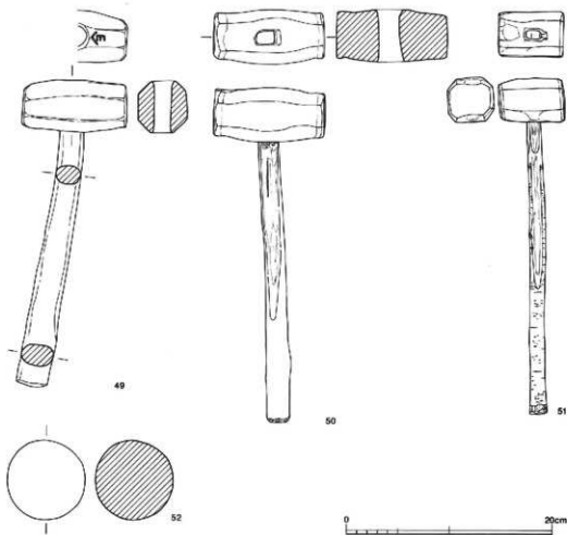
コブチ(49・50) コマヤタキ(51)
