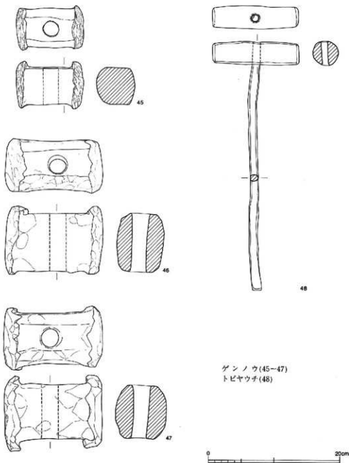
第21図 採石道具実測図(5)
