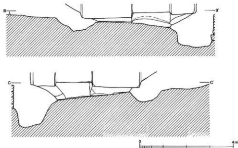
第27図 石宝殿 基部実測図
