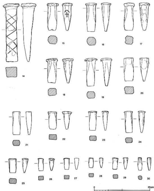
第19図 採石道具実測図(3)
