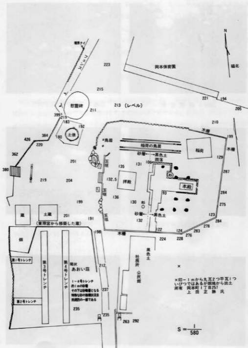
挿図8 辻が森三社境内礎石位置図
