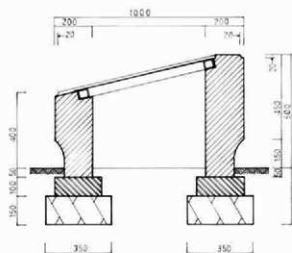
断面図 (1/20)
