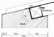
断面詳細図 (1/4)
