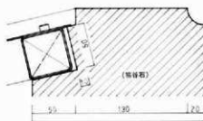
立面図 (1/20)
