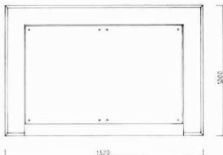
平面図 (1/20)
