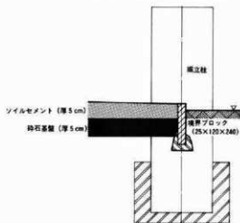
ソイルセメント舗装 (1/10)
