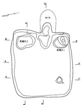
第37図 A区第13号住居跡
