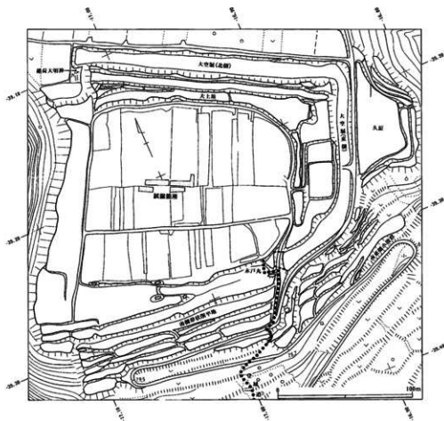
第11図 試掘溝設置箇所
