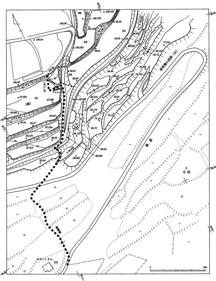
第10図 障ノ内館跡測量図④
