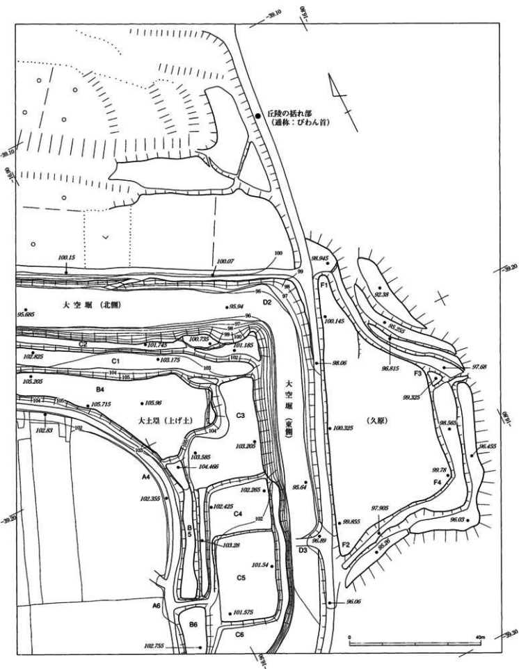
第8図 陣ノ内館跡測量図②
