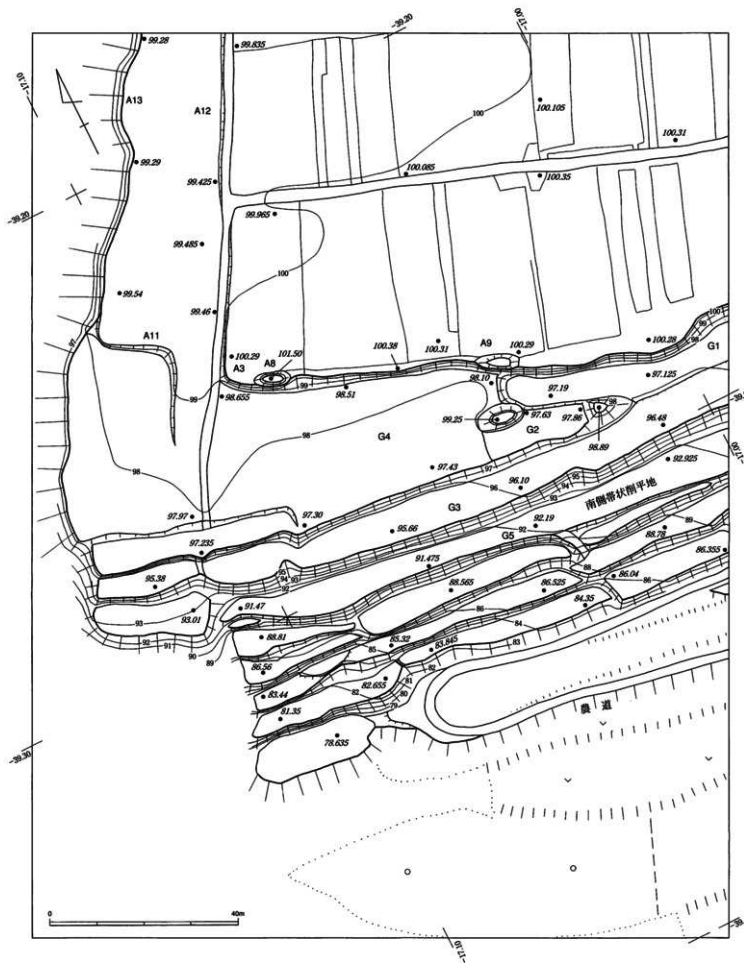
第9回 障ノ内館跡測量図③
