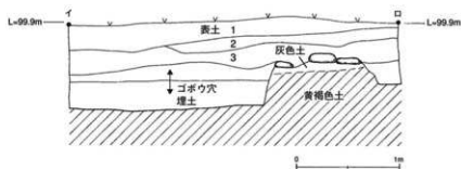
第12図 トレンチ西壁土層断面図
