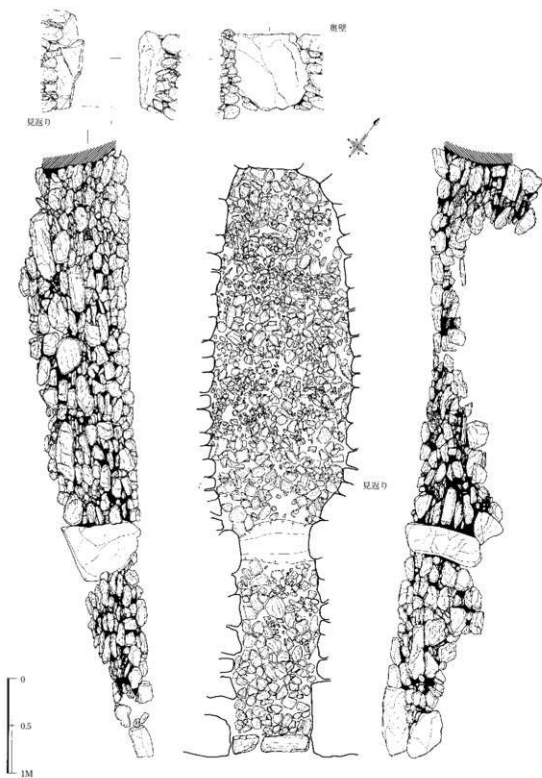
第17图 1号墳横穴式石室実測图 (S = 1/40)
