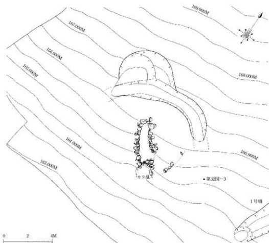
第25図 2号墳検出状況平面図 (S = 1/160)
