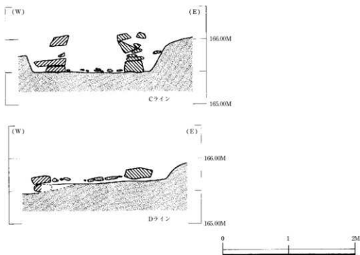
第28図 2号墳石室横断面 (S=1/40)
