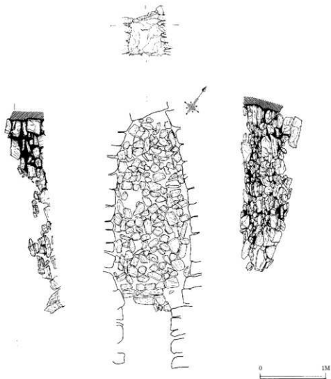
第27図 2号墳横穴式石室実測図 (S=1/40)
