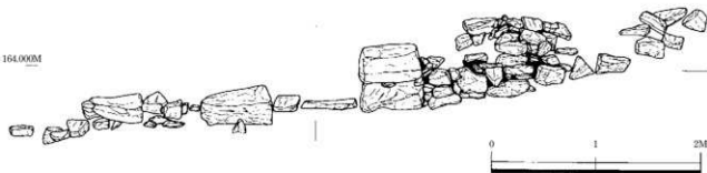
第18図 1号墳葺石立面図 (S=1/40)
