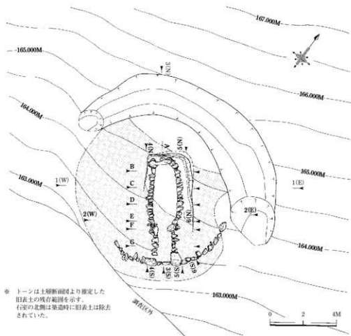
第22図 1号墳盛土撤去後 (S=1/160)
