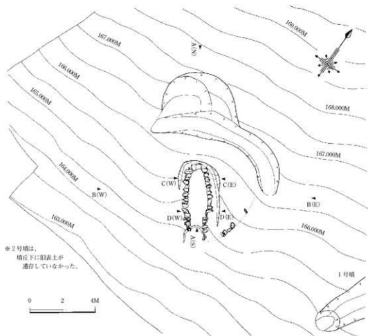
第31図 2号墳盛土撤去後 (S=1/160)
