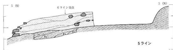
第20図 1号墳 墳丘断面図 (S=1/40)
