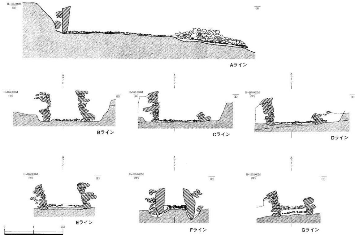
第21図 1号墳石室断面図 (S=1/40)
