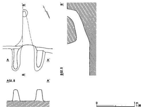
図46 石神境遺跡SI-22カマド平面図および断面図
