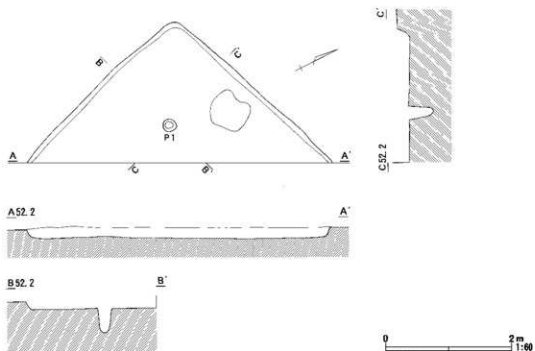
図27 石神境遺跡SI-12平面図および断面図
