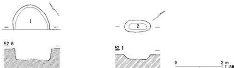
図48 石神境遺跡SK平面図および断面図
