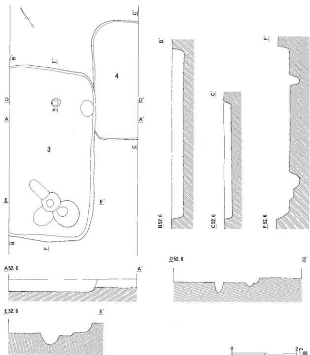
図9 石神境遺跡S1-3・4平面図および断面図
