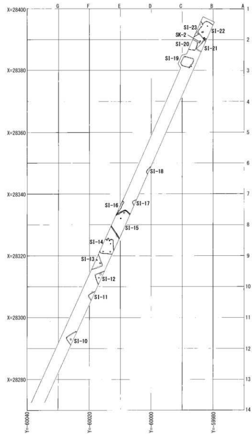
图4 石神境遺跡全体図
