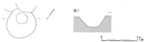
図10 石神境遺跡S1-3貯蔵穴平面図および断面図
