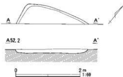
図38 石神境遺跡S1-18平面図および断面図
