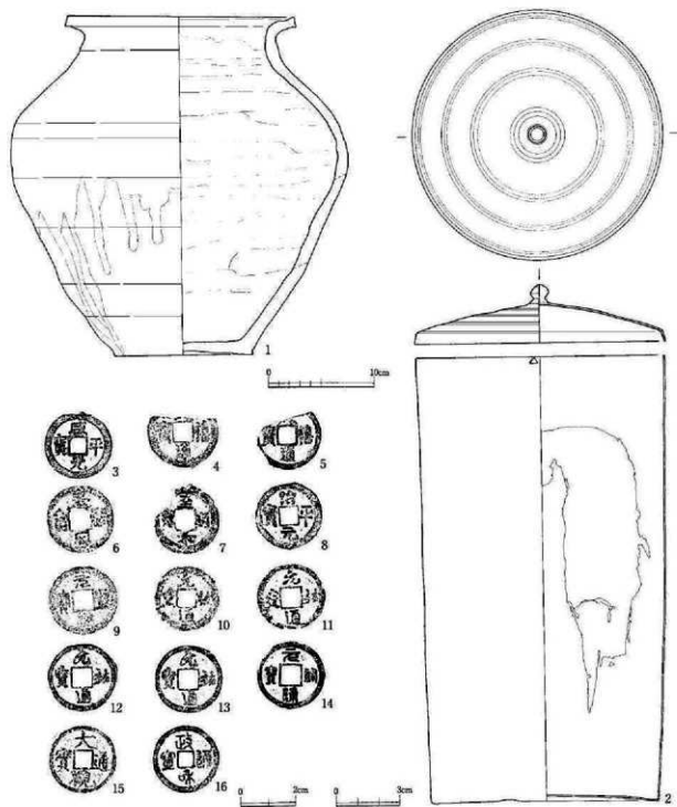
第20図 経塚2出土物実測図・拓影(1:縮尺1/4, 2:縮尺1/2, 3~16:縮尺2/3)
