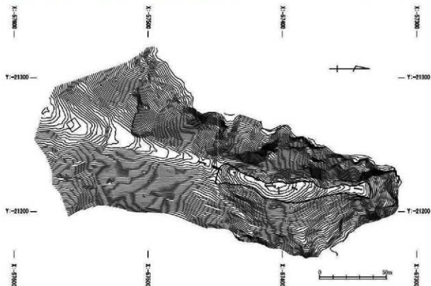
第4図 現況測量図(縮尺1/2,000) 西んだ部分が調査範囲
