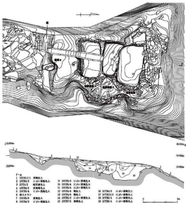
第9図 台状墓2実測図(縮尺1/100)
