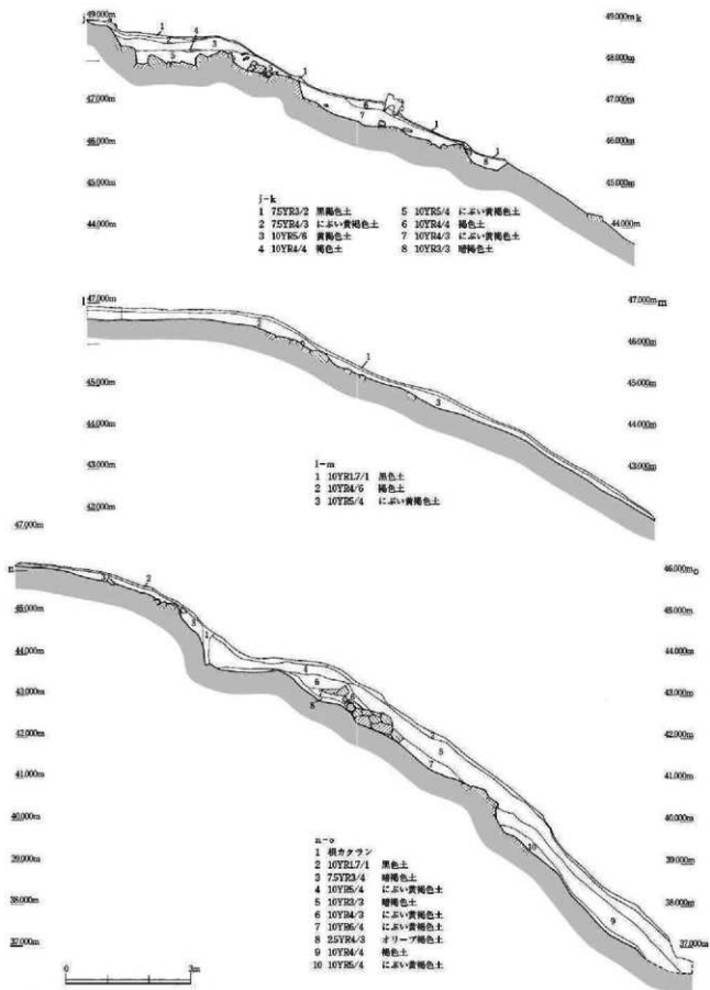
第23図 土層図2 (縮尺1/100)
