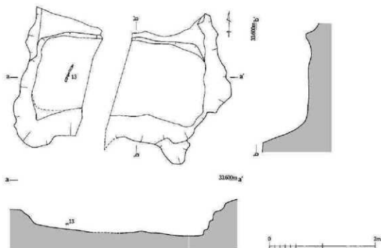
第12図 台状基2・埋葬施設3実測図(縮尺1/50) 图中的番号は第14図に対応
