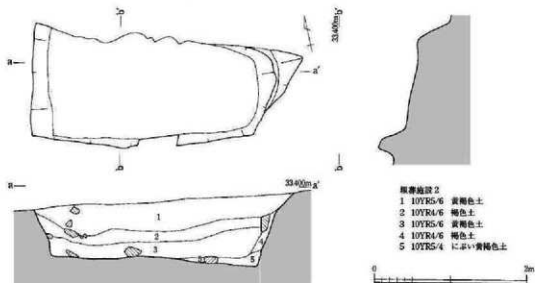
第11図 台状墓2・埋葬施設2実測図(縮尺1/50)
