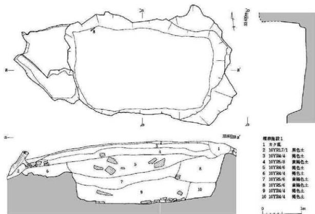
第10図 台状墓2・埋葬施設1実測図(縮尺1/50) 图中的番号は第13図に対応
