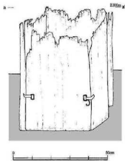
第32図 2区SE01実測図(縮尺1/10) 図中の番号は第33・34図に对应
