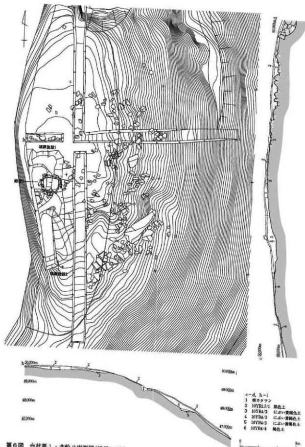
第6図 台状墓1・曲輪2実測図(縮尺1/100)
