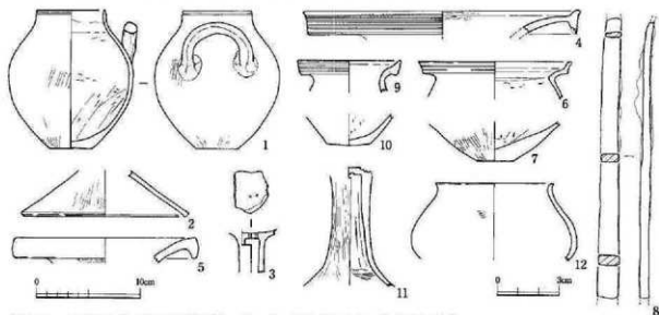
第13図 台状基2出土遺物実測図(1~7・9~12:縮尺1/4, 8:縮尺1/2)
