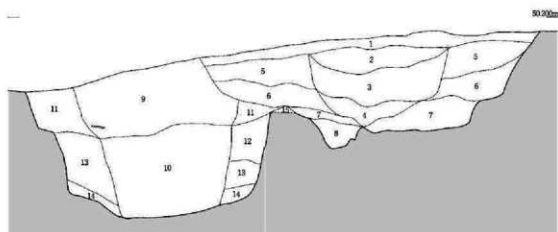
第7図 台状墓1・埋葬施設1・2実測図(縮尺1/50) 図中の番号は第8図に対応
