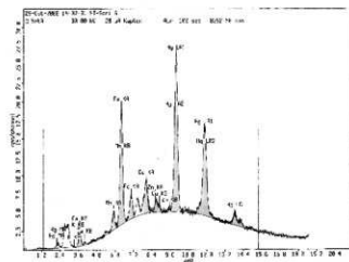
第269図 蛍光X線スペクトル (試料番号331)
