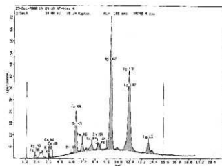
第268図 蛍光X線スペクトル (試料番号330)
