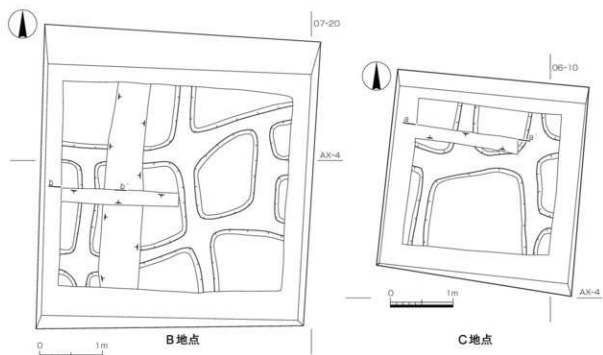
図35 B地点<7層>畦畔土層断面 (S=1/30)
