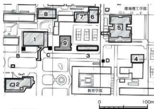
図4 調査地点の位置（A地点）（S=1/4,000）
