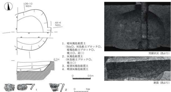
図31 SKc9 (S=1/30・1/4)
