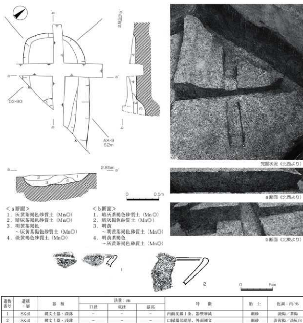
図49 SKd1・出土遺物 (S=1/30・1/4)
