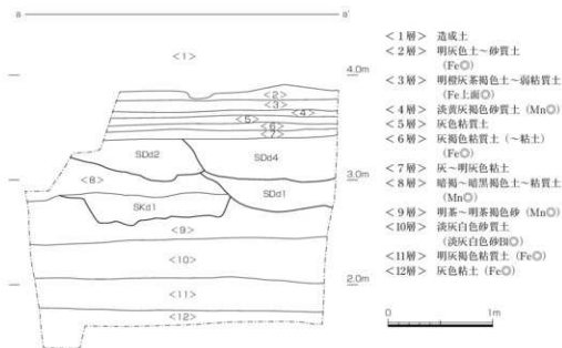
図46 土層断面（南壁）(S=1/40)
