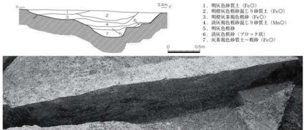
図58 SDd4断面 (S=1/30)
