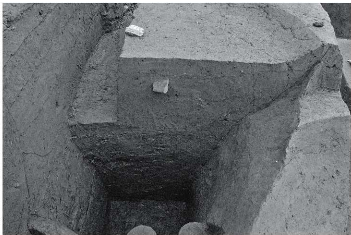
2. 土層断面 (南から)
