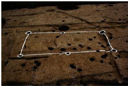
3 第 15 号掘立柱建物
