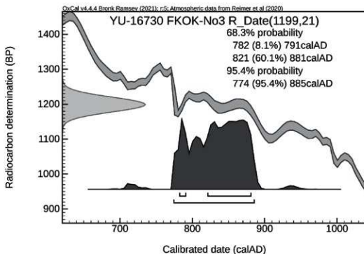
図1 Ⅶ区003号区遺構計測結果
