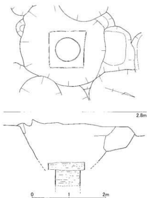
Fig.190 ⅩⅨ区357号遺構実測図(1/50)
