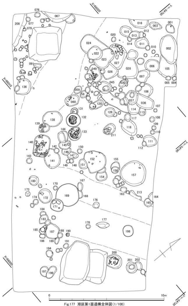
Fig.177 邺区第1面遗構全体圖(1/100)
