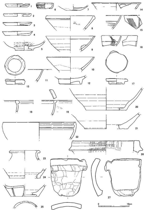
Fig.188 邙区342号遗址出土遗物实测图(1/3)
