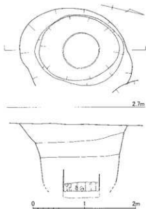
Fig.187 Ⅹ区342号遺構実測図(1/50)
