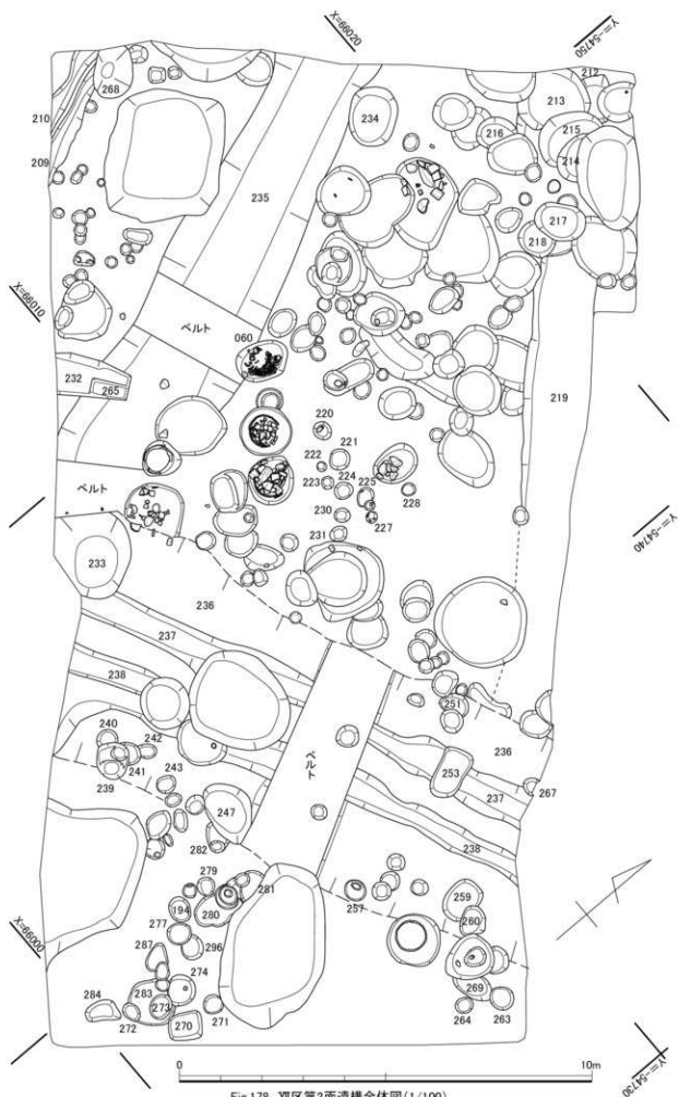
Fig.178 Ⅱ区第2面遺構全体圖(1/100)
