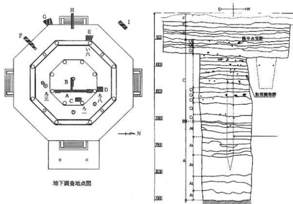
図4 西大寺東塔基壇の断面と銅銭出土位置 1:70 (奈良研 1982『奈良国立文化財研究所年報 1982』)
