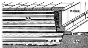
図3 基壇版築と地覆地業模式図
