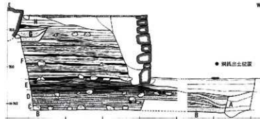
図4 西大寺東塔基壇の断面と銅銭出土位置 1:70 (奈良研 1982『奈良国立文化財研究所年報 1982』)
