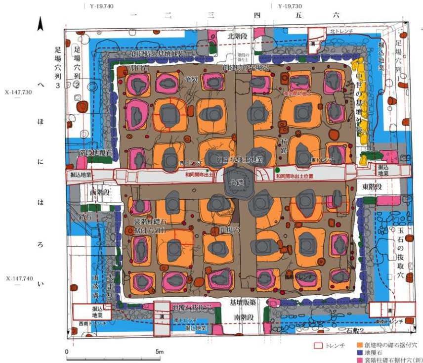
図1 調査区平面図 1:100
