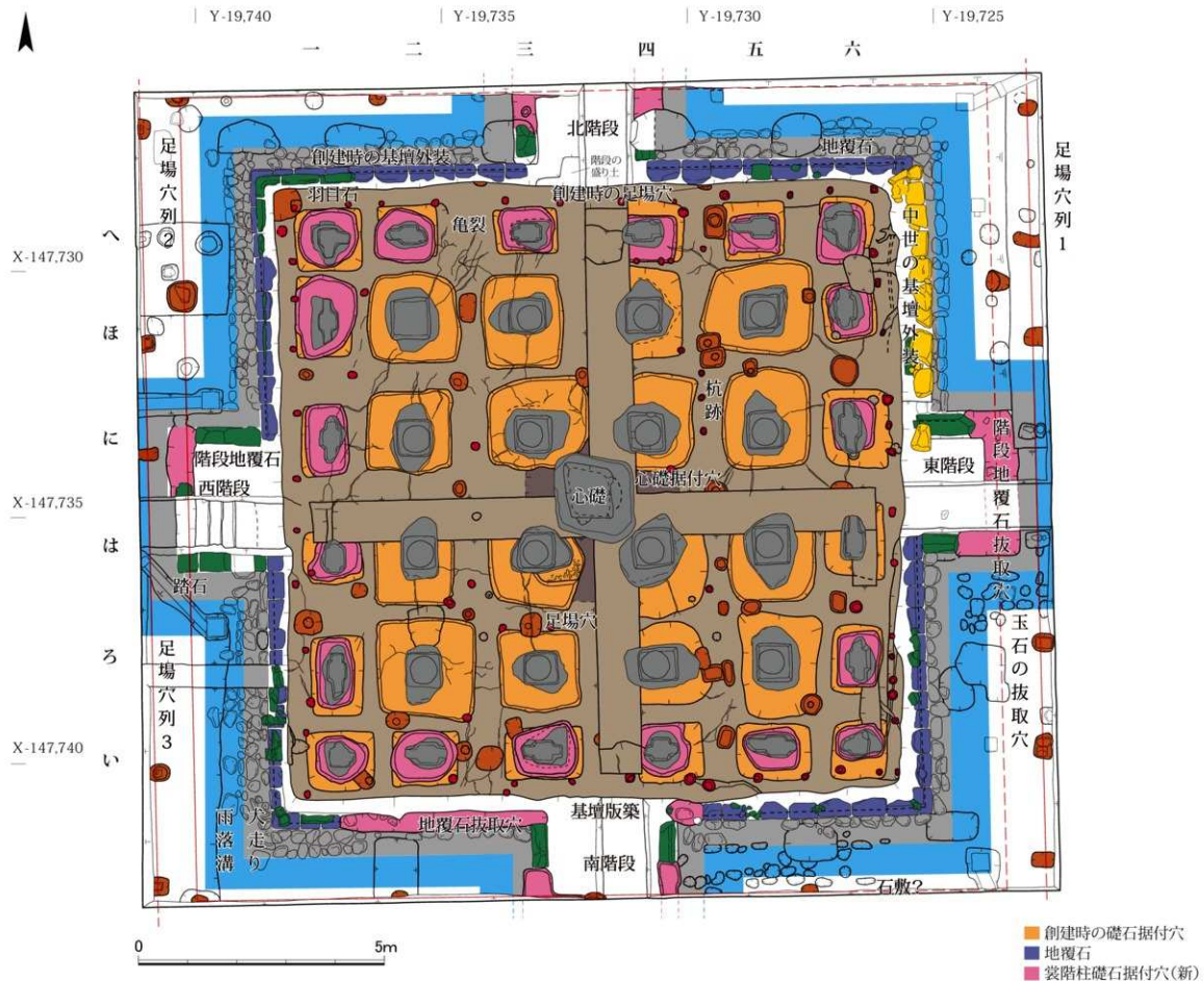
図7 調査区平面図 1:80
