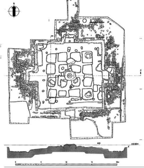
【参考】薬師寺西塔平面・断面図
