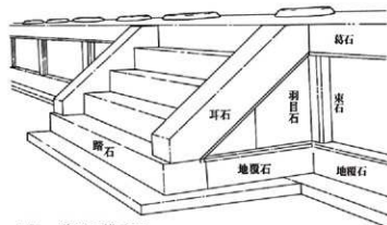
図5 階段の模式図
