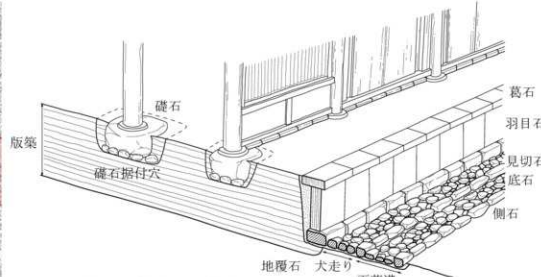
図4 基壇および基壇周囲の模式図
