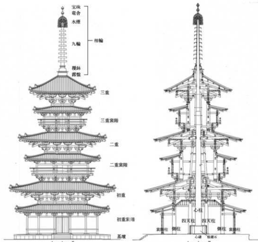
図3 東塔の各部名称
