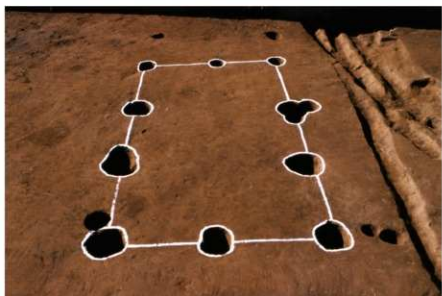
2 第7-2号掘立柱建物跡
