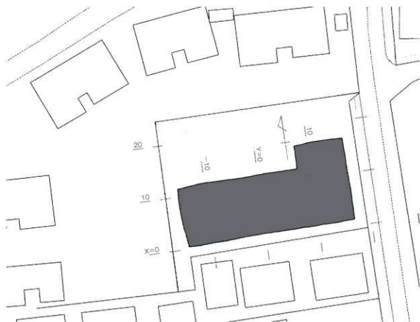
图4 调查区位置图 (S = 1 / 500)
