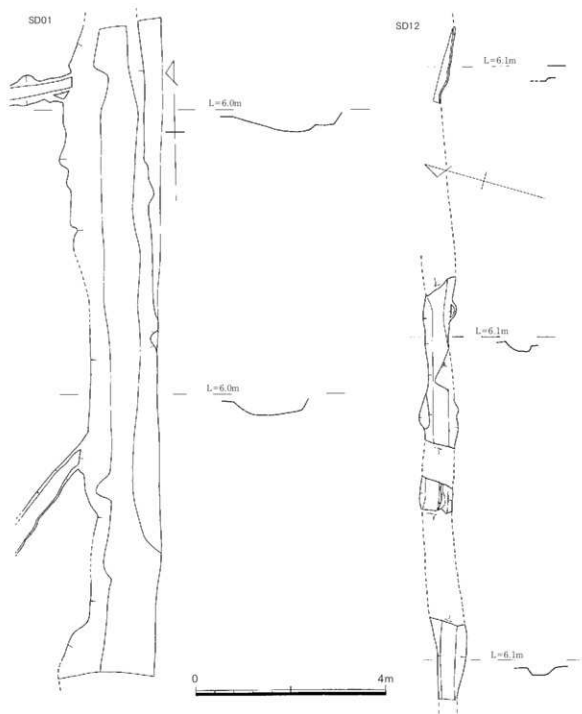
図6 SD01・12実測図 (S = 1/80)
